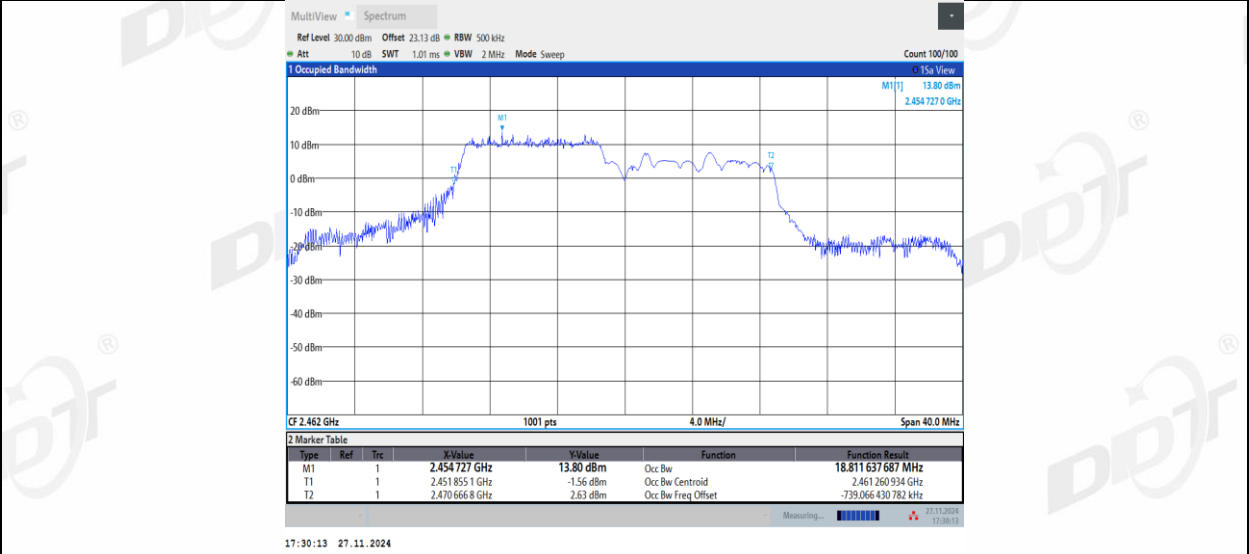
11AX20MIMO_Ant1_2462_106Tone_RU54
