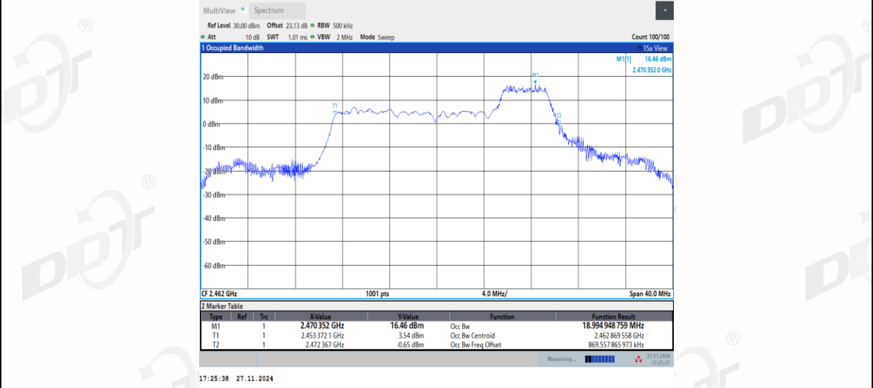
11AX20MIMO_Ant1_2462_106Tone_RU53
