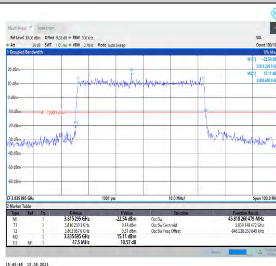
1-N77-3700-3980-PC1-30-50-M-4-DFT-64QAM-Out er Full-128@0-Ant0-45.818-47.500-≤50-PASS
