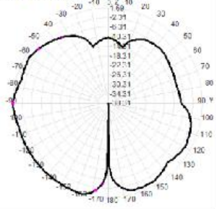
2470.0MHz Total(E2-YZ), Max= 1.69dBi
