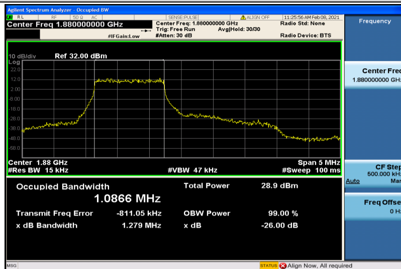
Band2-3MHz-QPSK-18900-6RB#0-1.0866
