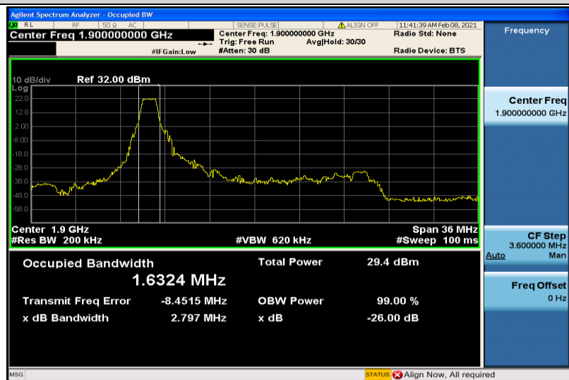
Band2-20MHz-QPSK-19100-6RB#0-1.6324
