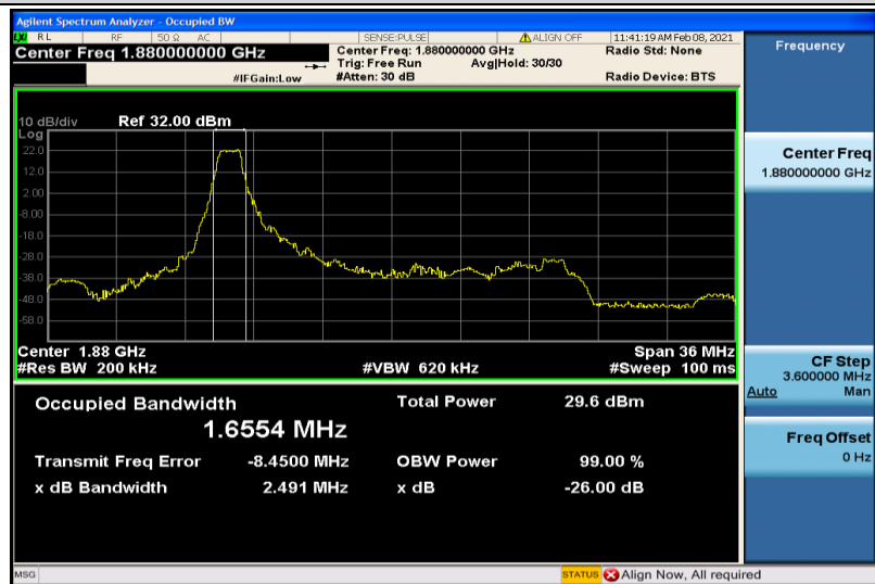
Band2-20MHz-QPSK-18900-6RB#0-1.6554
