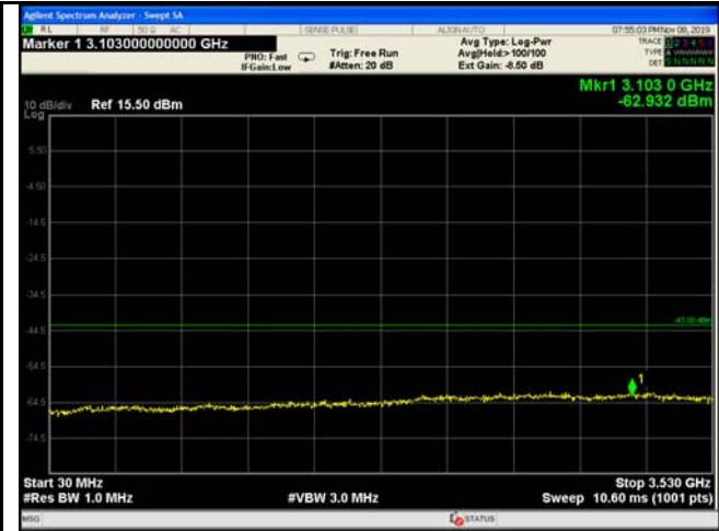
5MHz - Low CH 30MHz~3.53GHz
