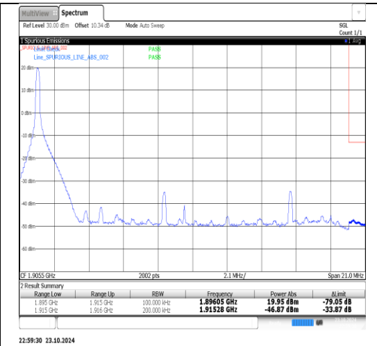
Band25-20MHz-QPSK-26590-1RB#99-PASS
