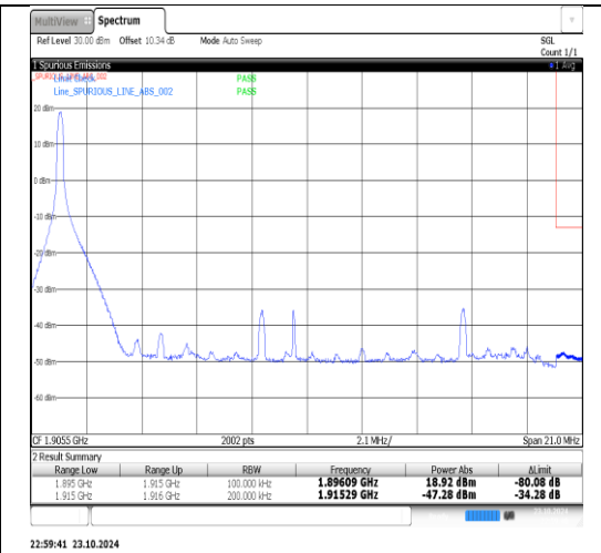
Band25-20MHz-16QAM-26590-1RB#99-PASS
