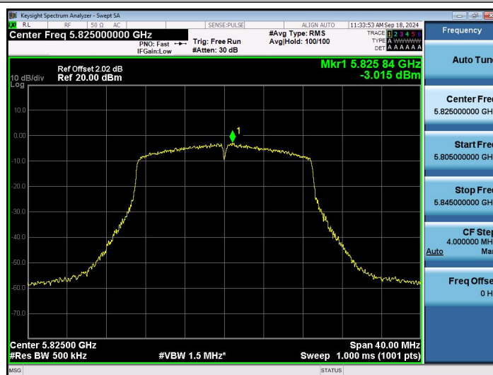
802.11n(HT20)SISO-Ant1-5825-PASS
