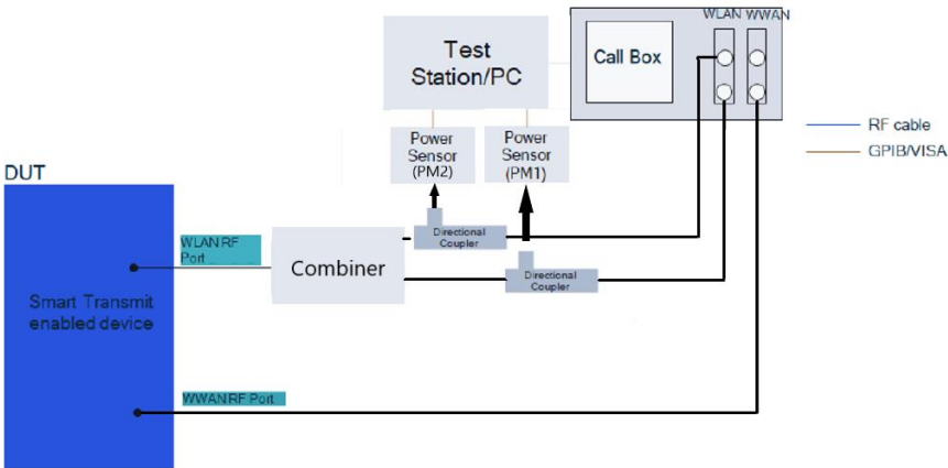
(d) Appendix A – Test Setup Photo 6
