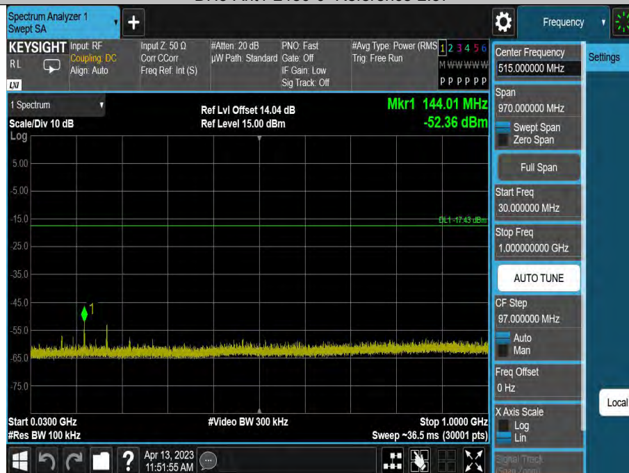
DH5-Ant1-2480-30~1000-2.57
