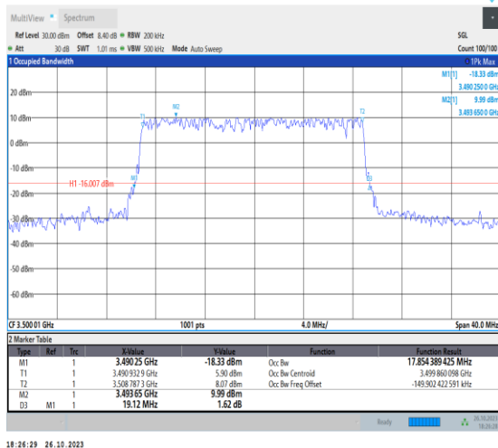
1-N78-3450-3550-PC2-30-20-M-5-DFT-256QAM-Outer_Full-50@0-Ant0-17.854-19.120-≤20-PASS
