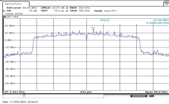
11BE20-CDD_Ant1_2437_0~Reference
