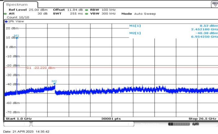
11BE20-CDD_Ant3_2457_1000~26500
