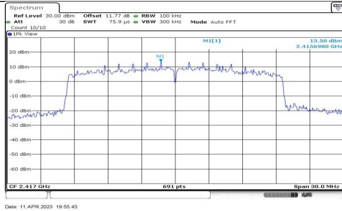
11BE20-CDD_Ant4_2417_0~Reference
