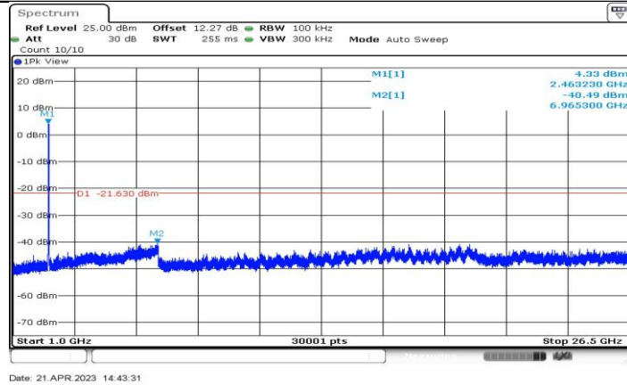
11BE20-CDD_Ant2_2462_1000~26500
