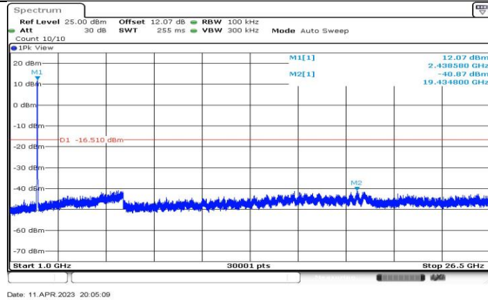
11BE20-CDD_Ant1_2437_1000~26500
