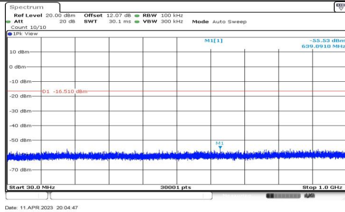
11BE20-CDD_Ant1_2437_30~1000
