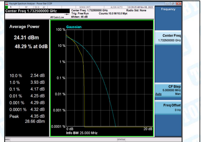
Band4-20MHz-QPSK-20175-1RB#0-PASS
