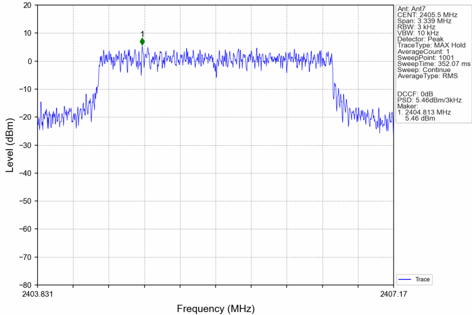
3M_LCH_2405.5MHz_MIMO_NTNV
