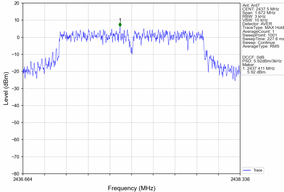
1.4M_MCH_2437.5MHz_MIMO_NTNV
