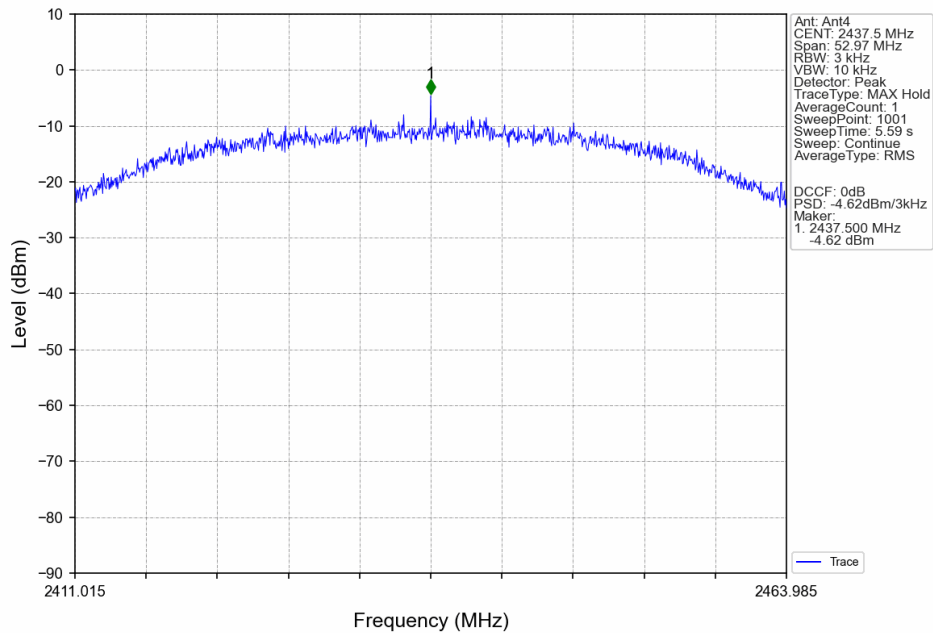
60M_MCH_2437.5MHz_Ant4_NTNV
