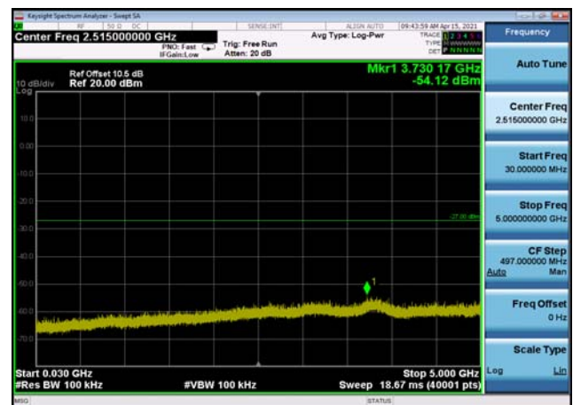
U-NII-3 ,Plot 2,30MHz~5000MHz-802.11a (20MHz),5745MHz,Ant1
