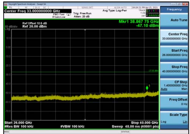
U-NII-3 ,Plot 2,26000MHz~40000MHz-802 .11ac(40MHz),5755MHz,Ant1
