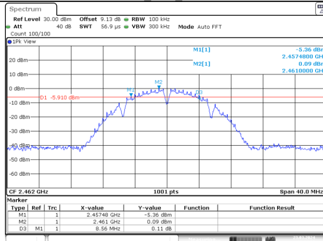
11B_Ant1_2462
