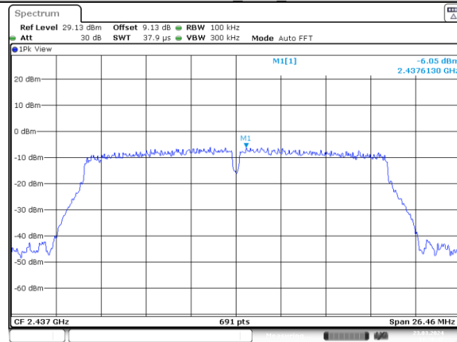
11N20SISO_Ant1_2437
