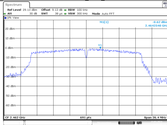
11N20SISO_Ant1_2462
