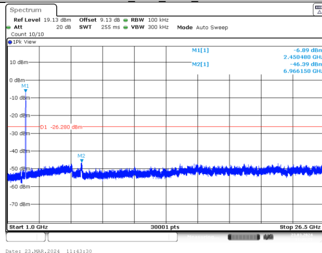
11N40SISO Ant1 2452 1000~26500
