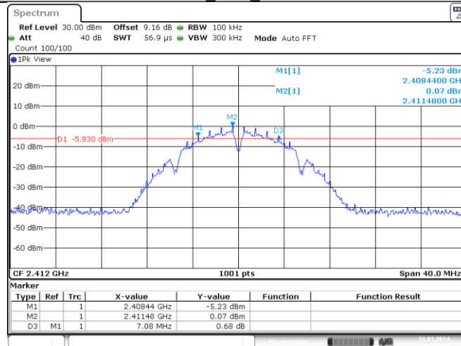
11B_Ant1_2412
