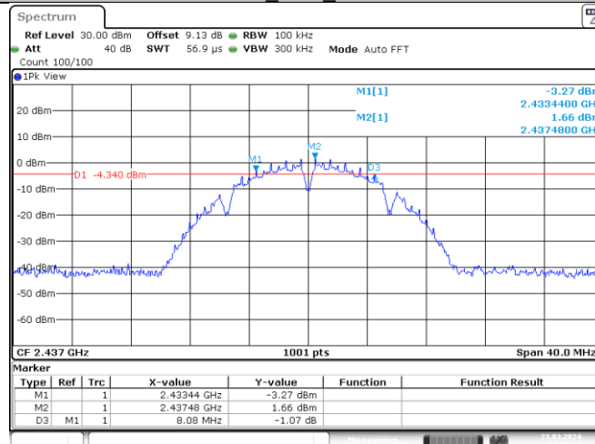
11B_Ant1_2437
