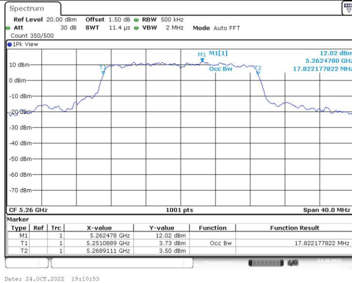
11AC20MIMO_Ant2_5260
