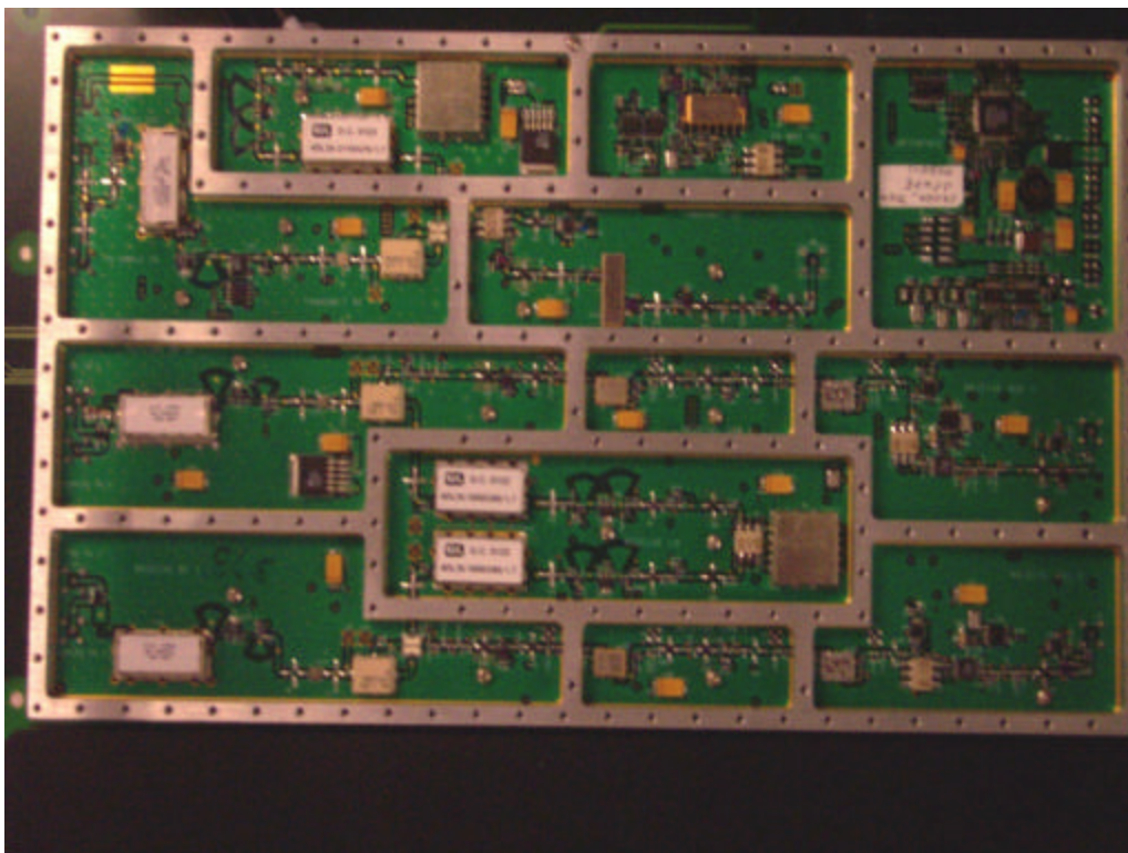
RAS front Model:RM-1900 800002 FCC ID: QHY800002
