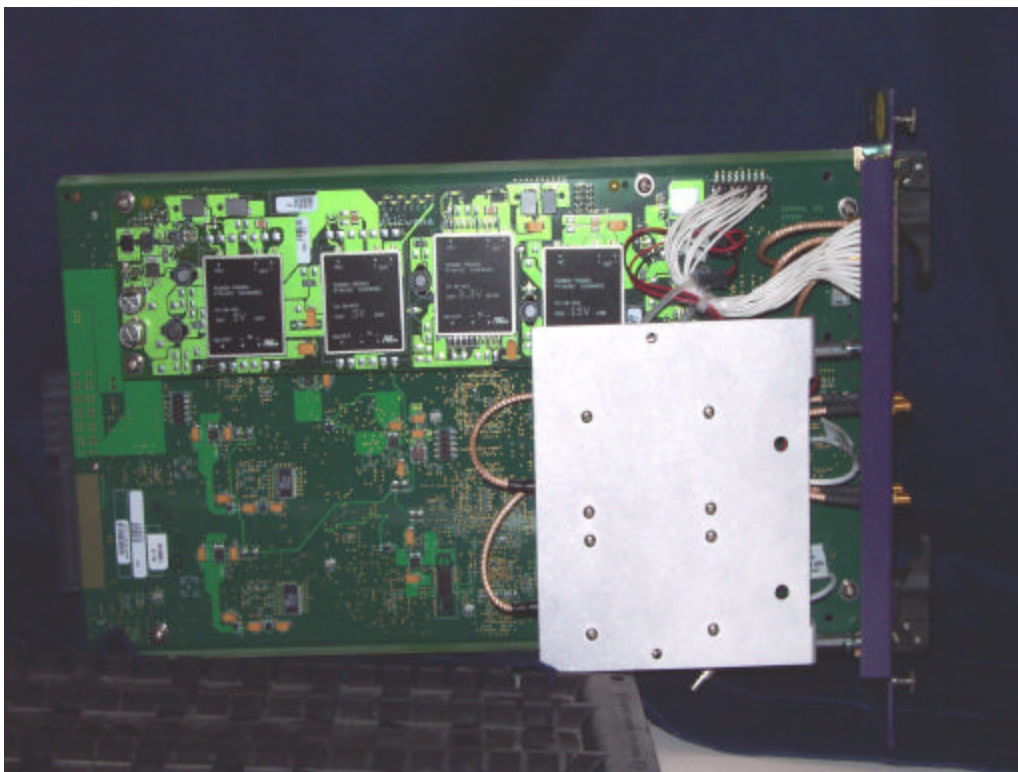
Radio Module Left Side Model:RM-1900 800002 FCC ID: QHY800002
