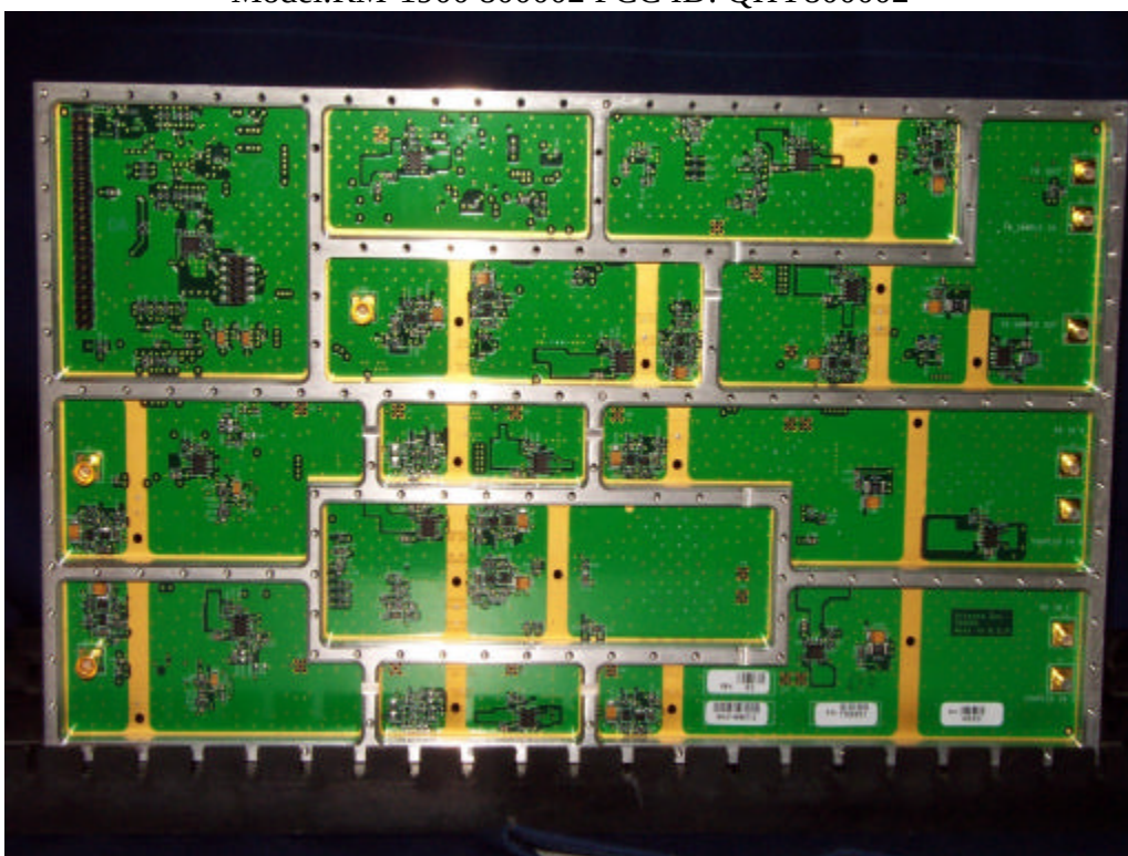
RAS back Model:RM-1900 800002 FCC ID: QHY800002
