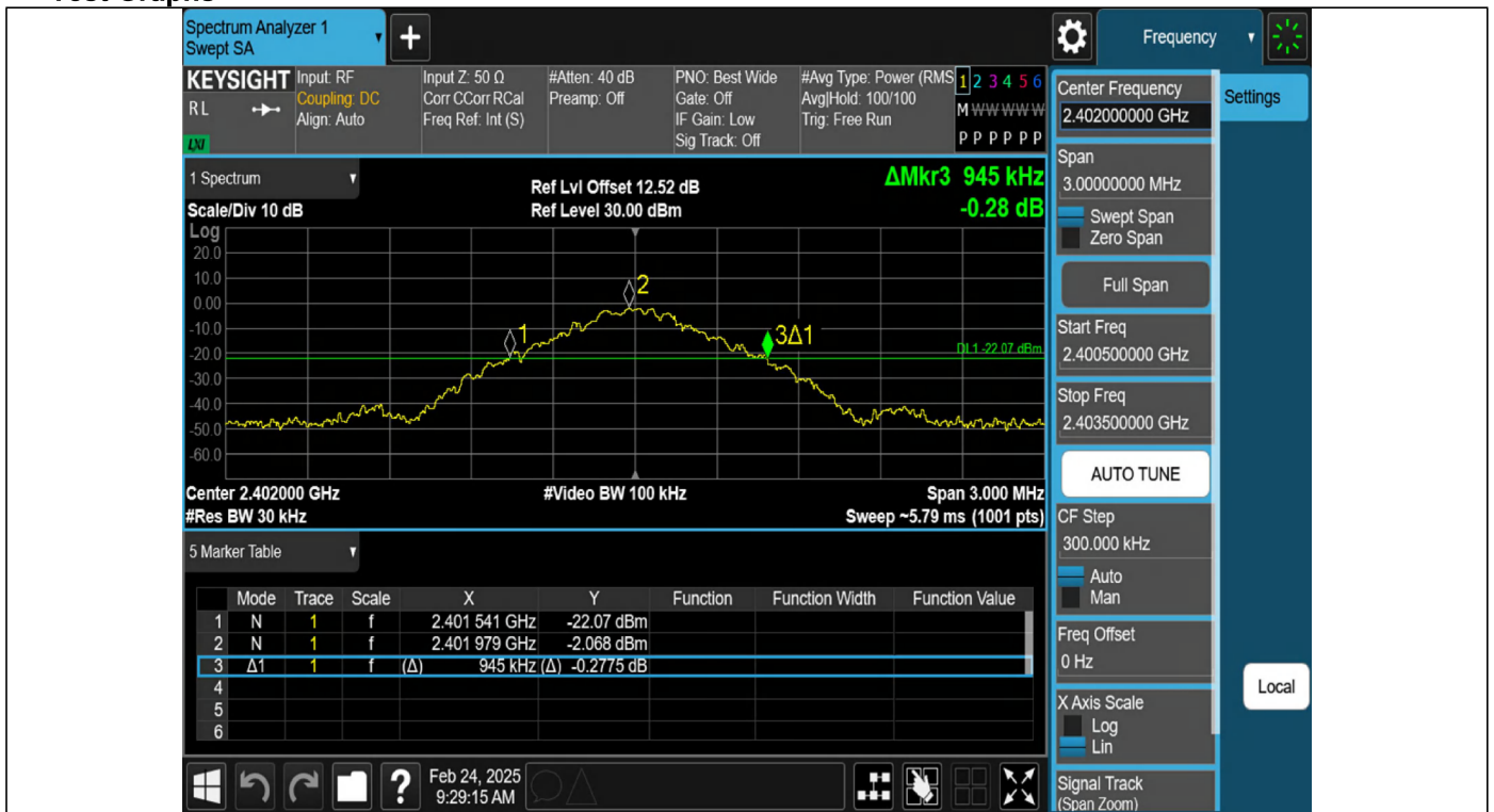
DH5-Ant1-2402
