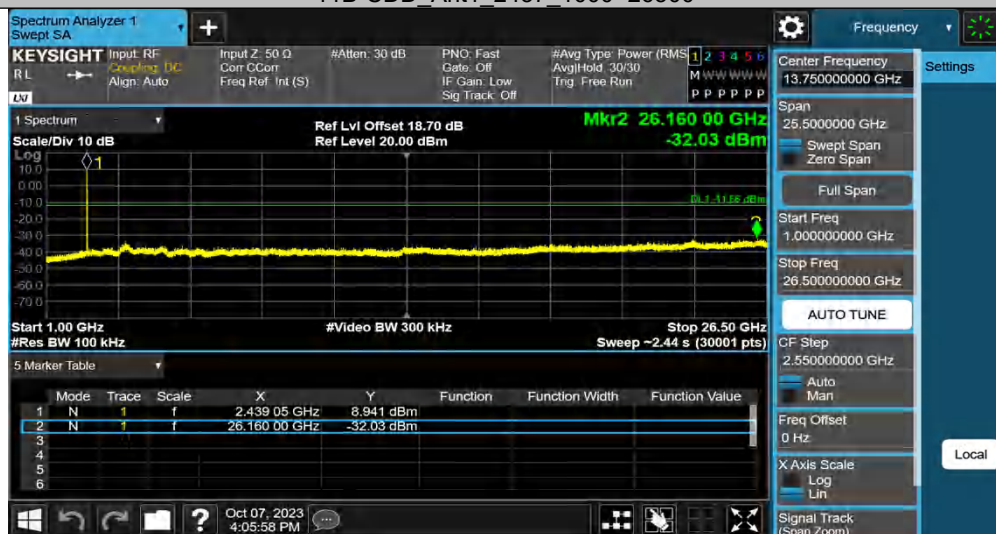
11B-CDD_Ant1_2462_0~Reference
