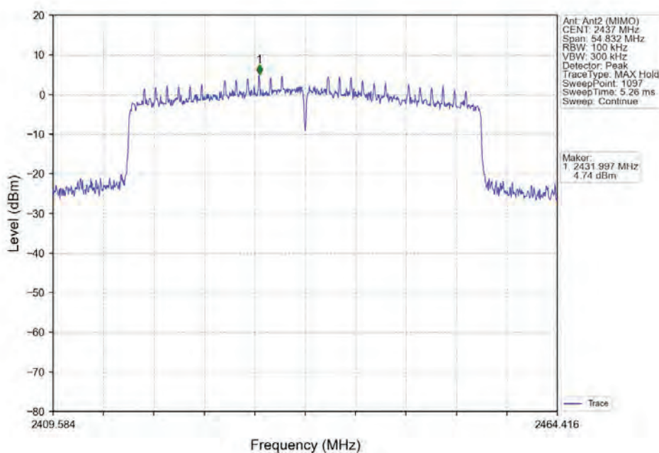
802.11ax(HEW40)_MCH_2437MHz_RU484_Left_Ant2 (MIMO)_NTNV
