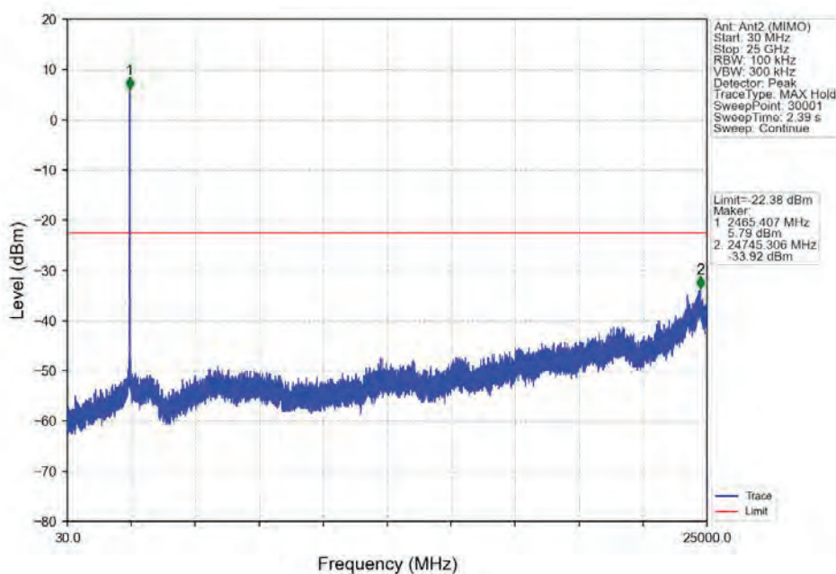
802.11ax(HEW20)_HCH_2462MHz_RU242_Left_Ant2 (MIMO)_NTNV
