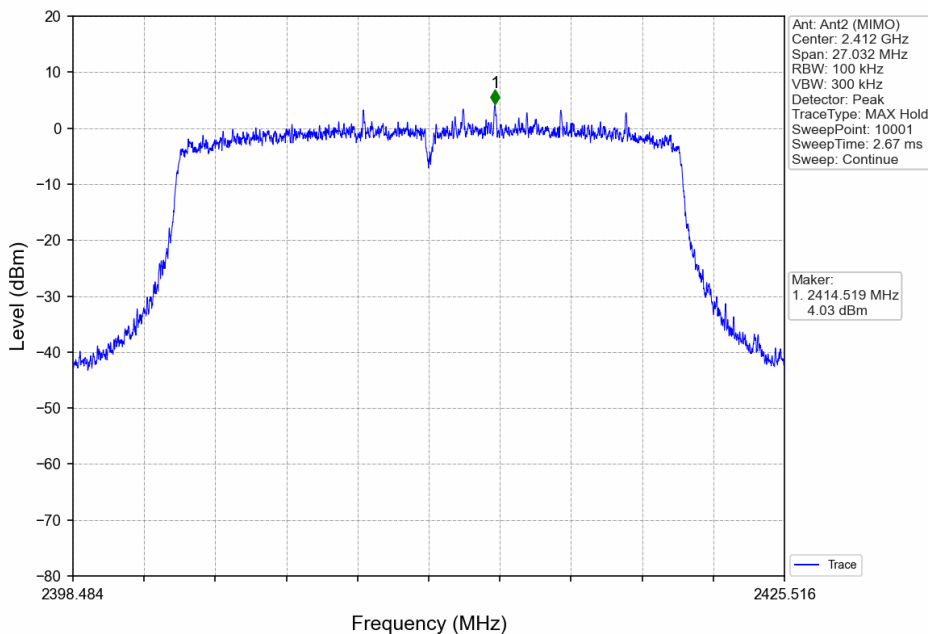
802.11ax(HEW20)_LCH_2412MHz_RU242_Left_Ant2 (MIMO)_NTNV
