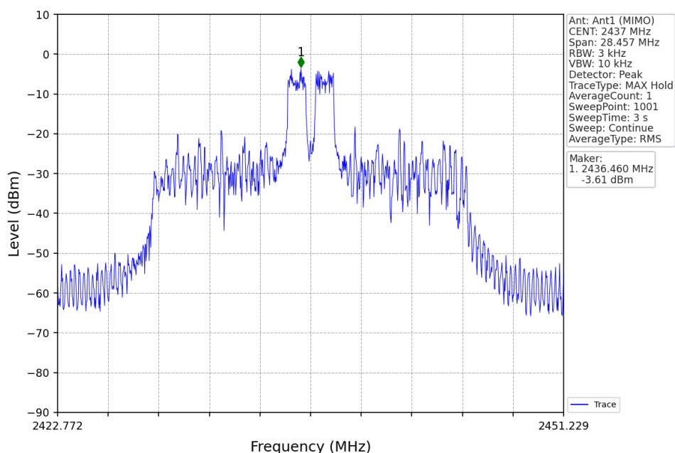
802.11ax(HEW20)_MCH_2437MHz_RU26_Mid_Ant1 (MIMO)_NTNV
