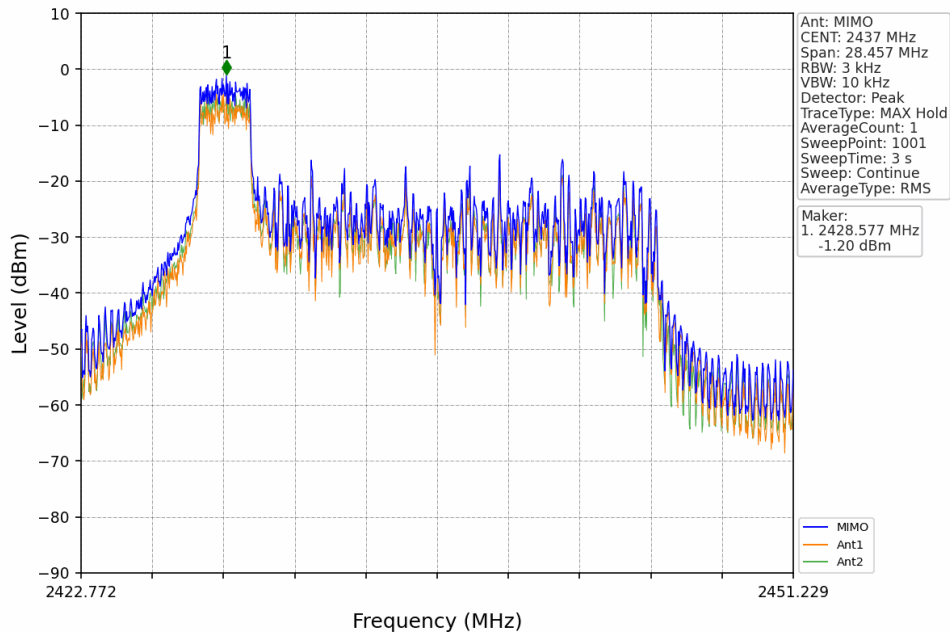
802.11ax(HEW20)_MCH_2437MHz_RU26_Mid_Ant1 (MIMO)_NTNV
