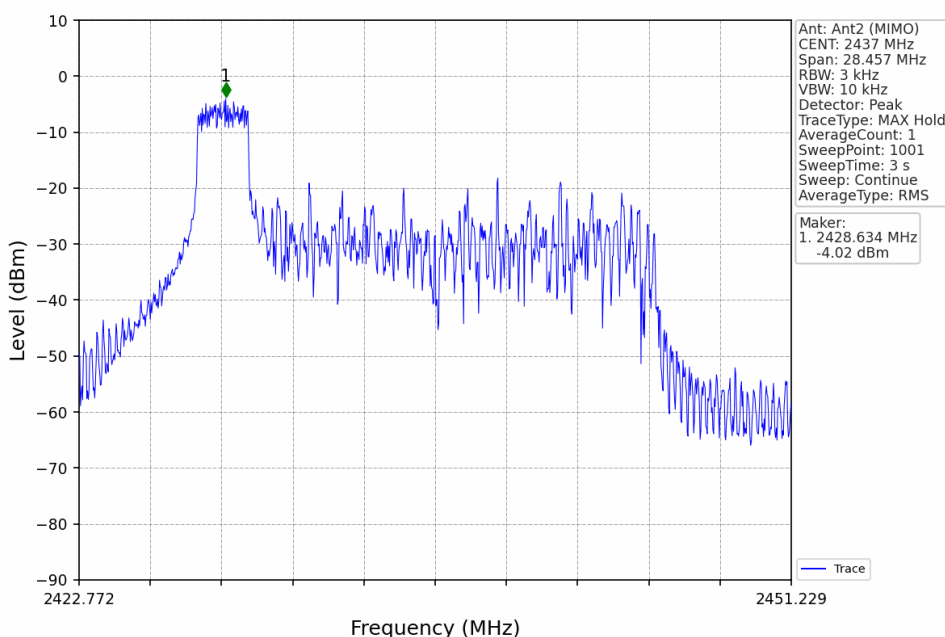
802.11ax(HEW20)_MCH_2437MHz_RU26_Left_Ant2 (MIMO)_NTNV
