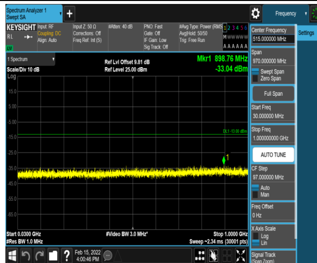
Band25-5MHz-QPSK-26365-1-0-Low-30-1000--33.04-PASS
