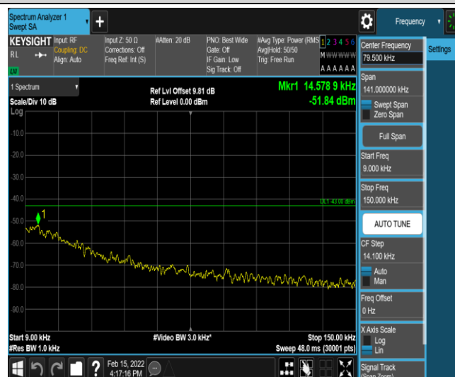
Band25-10MHz-QPSK-26365-1-0-Low-0.009-0.15--51.84-PASS
