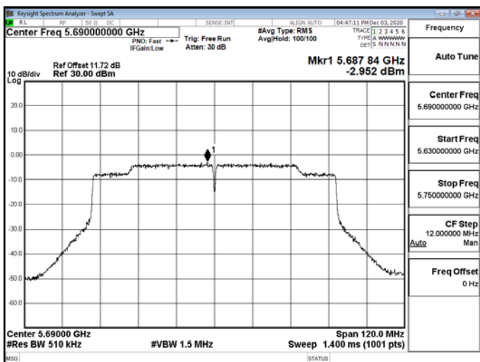
802.11ac_80MHz_CH0_5690MHz_UNII 3
