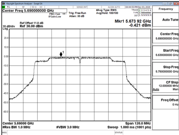
802.11ac_80MHz_CH1_5690MHz_UNII 3
