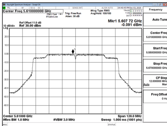
802.11ac_80MHz_CH1_5610MHz-5610
