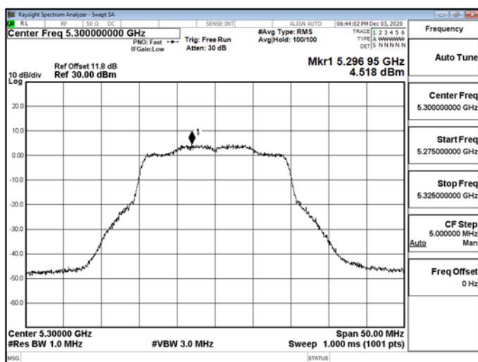
802.11ax_20MHz_CHO_5300MHz-5300
