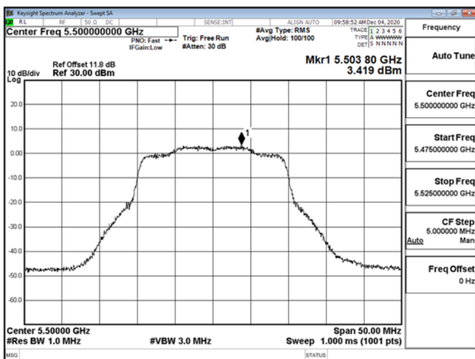
802.11ax_20MHz_CH1_5500MHz-5500
