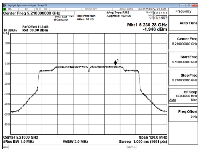
802.11ac_80MHz_CH1_5210MHz-5210
