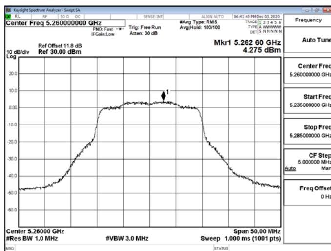
802.11ax_20MHz_CH1_5260MHz-5260
