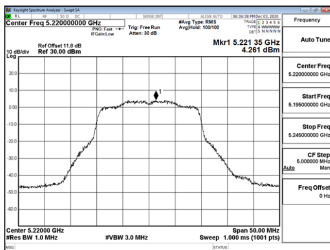
802.11ax_20MHz_CH0_5220MHz-5220
