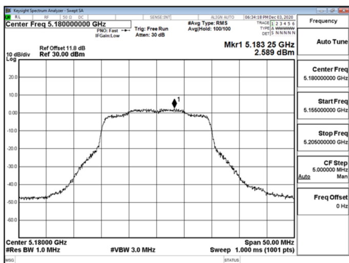
802.11ax_20MHz_CH1_5180MHz-5180
