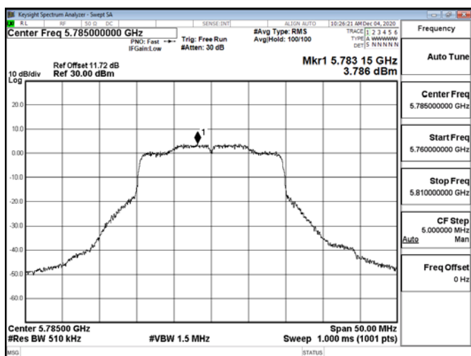
802.11ax_20MHz_CH1_5785MHz-5785
