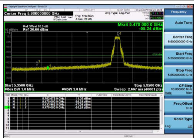
U-NII-2c ,Plot 1,Band Edge-802.11ac(20 MHz),5700MHz,Ant1
