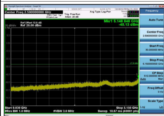
U-NII-1 ,Plot 2,30MHz~5150MHz-802.11a c(20MHz),5220MHz,Ant1
