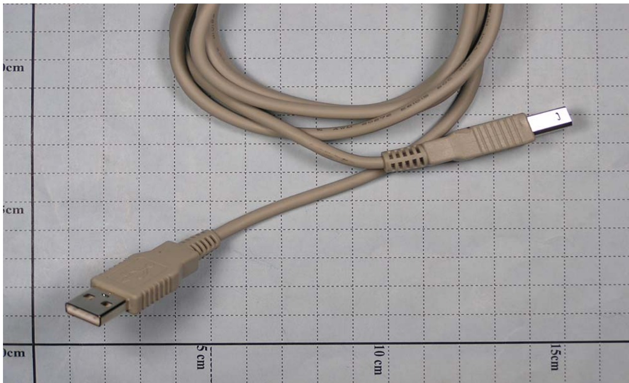
DATA/PWR CABLE
