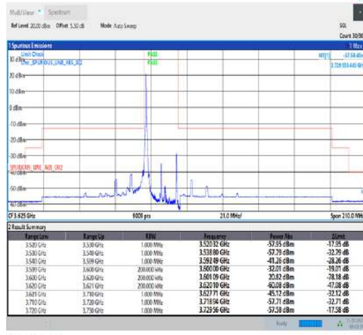
Band43_20MHz_QPSK_43690_1RB#0
