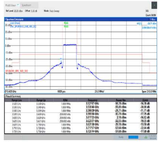
Band43_20MHz_QPSK_43690_100RB#0
