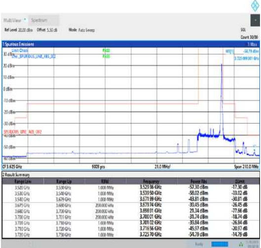
Band43_20MHz_QPSK_43690_1RB#0
