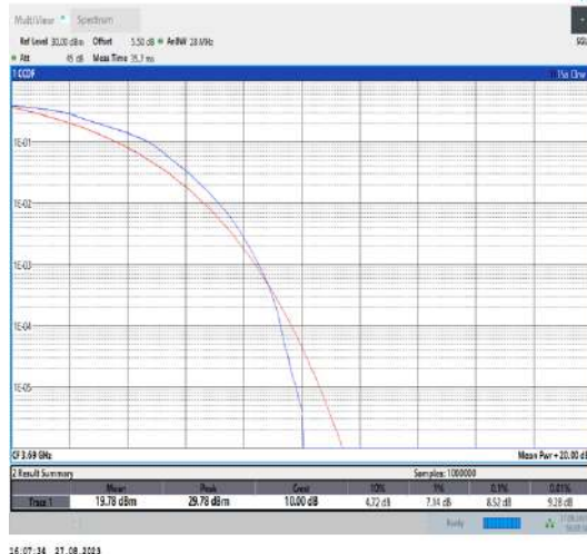
Band43-20MHz-16QAM-44490-100RB#0-PASS
