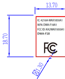
X-1850 下蓋銘版尺寸
