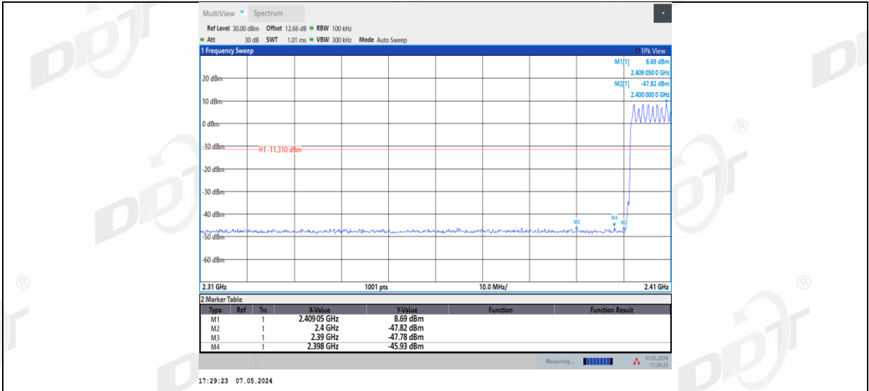
2DH5_Ant2_R_Low_Hop_2402
