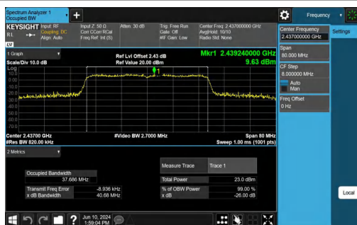
11AX40ISO-Ant1-2437
