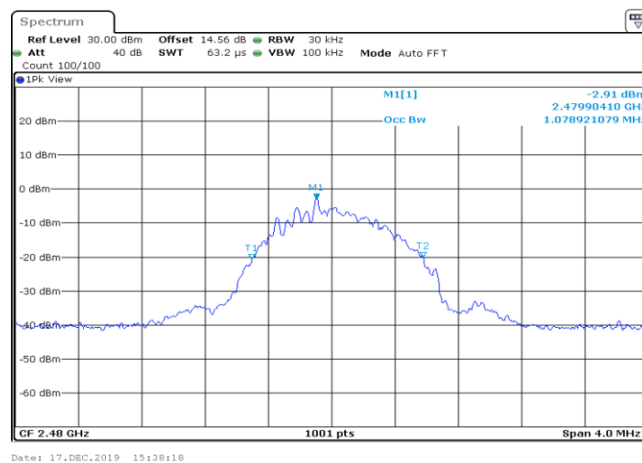
BLE_BT4.0_Ant1_2480
