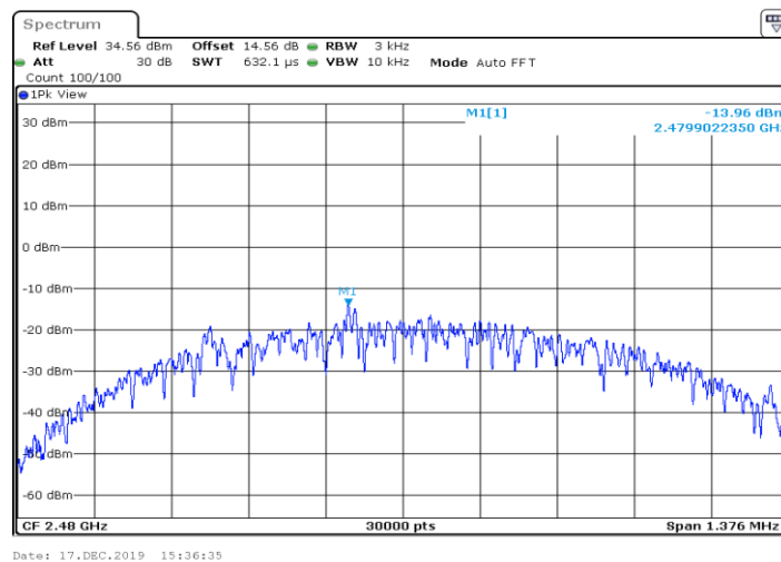
BLE_BT4.0_Ant1_2480
