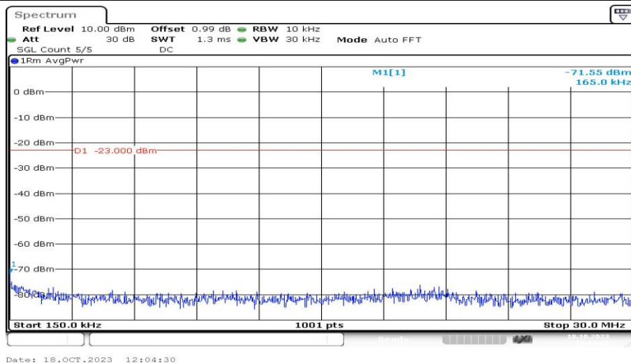
Band4-1.4MHz-QPSK-20393-1RB#0-Range2:0.15~30MHz-PASS
