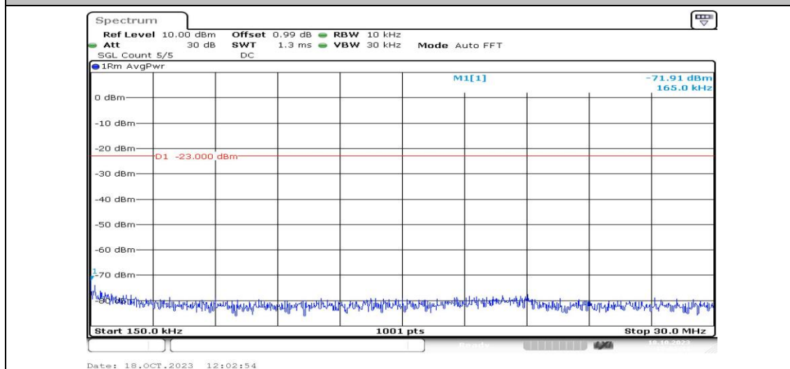
Band4-1.4MHz-QPSK-20175-1RB#0-Range2:0.15~30MHz-PASS
