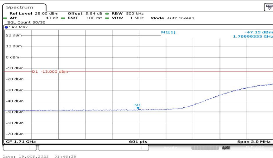
Band4-20MHz-16QAM-20050-1RB#99-PASS
