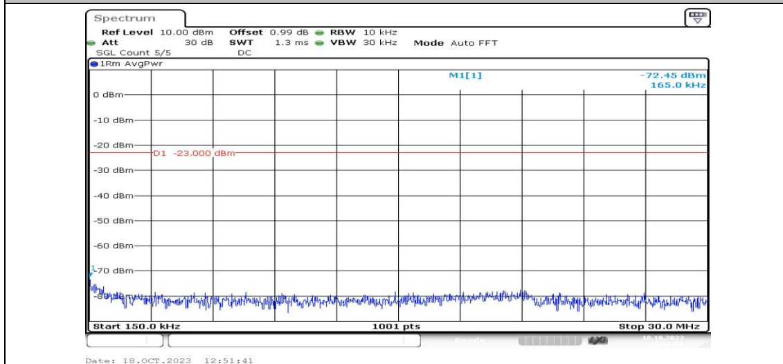
Band4-5MHz-QPSK-20175-1RB#0-Range2:0.15~30MHz-PASS
