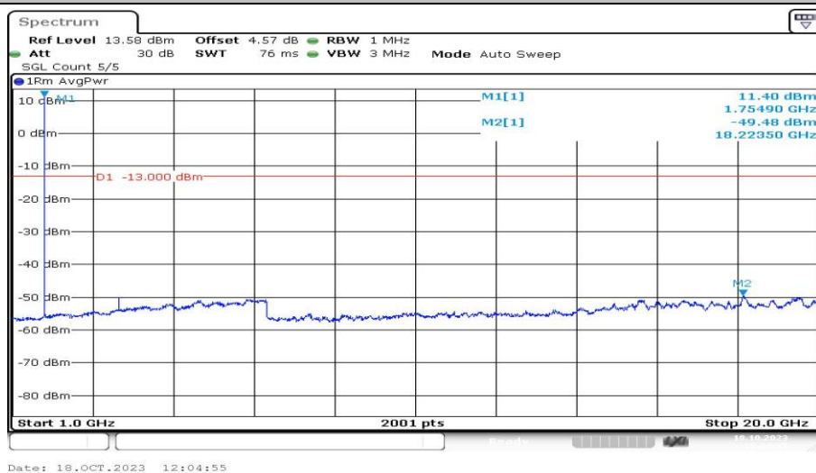
Band4-1.4MHz-QPSK-20393-1RB#0-Range4:1000~20000MHz-PASS
