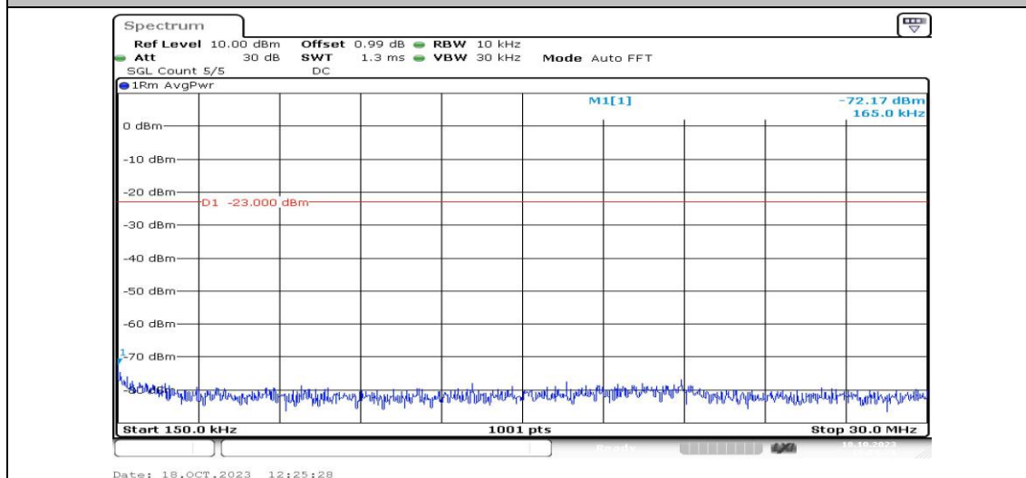
Band4-3MHz-QPSK-19965-1RB#0-Range2:0.15~30MHz-PASS
