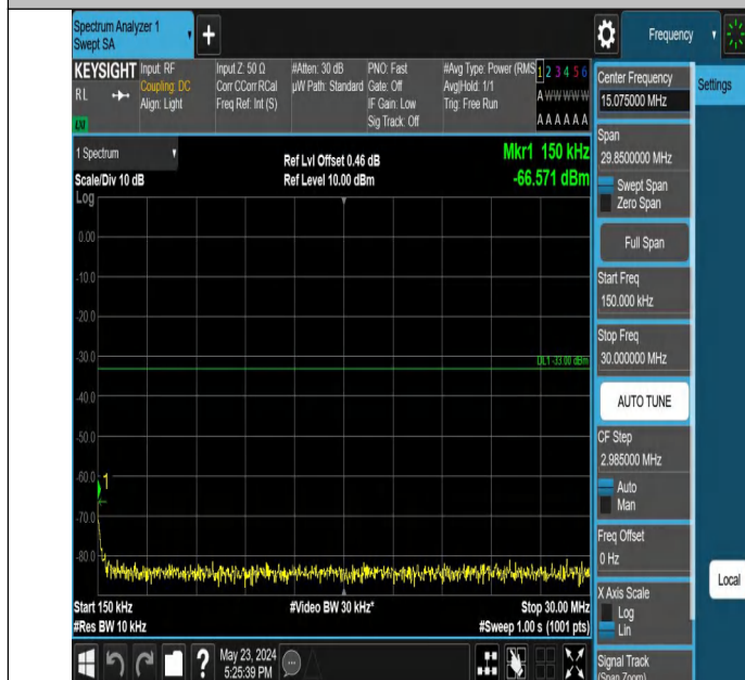
Band2 10MHz QPSK 18900 1RB#49 0.15~30 0.15~30
