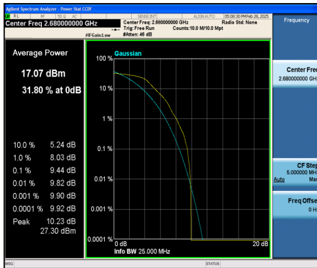
Band41-20MHz-QPSK-41490-1RB#0-PASS
