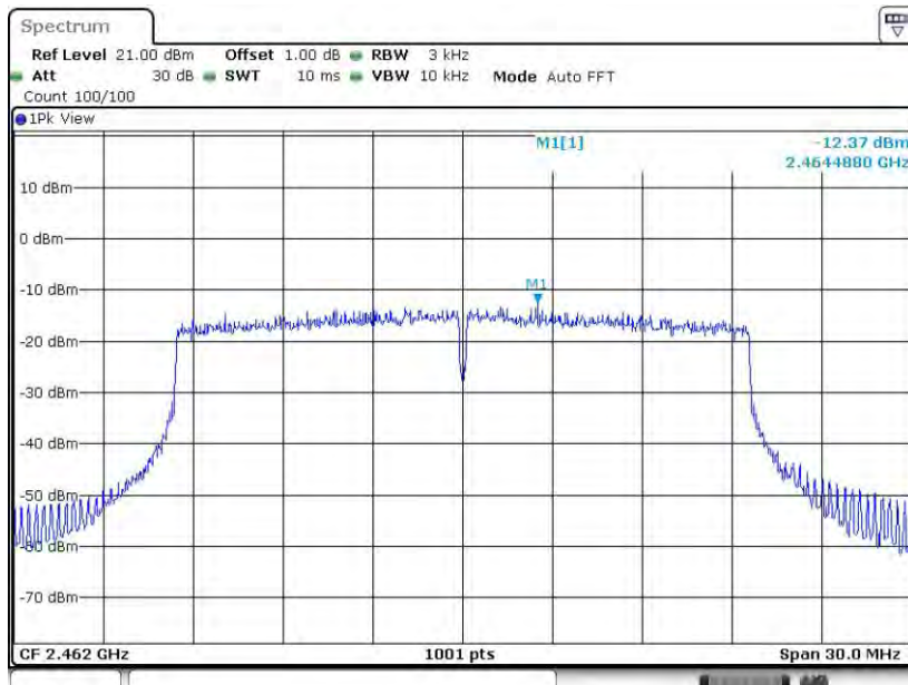
11AX20SISO_Ant7_2462
