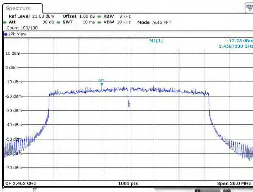
11AX20SISO_Ant2_2462
