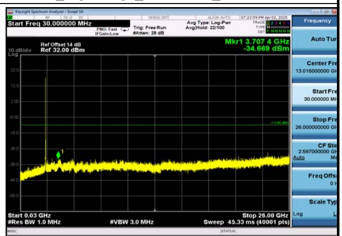
FDD7_MiddleRange_20+10MHz_30MHz~26GHz
