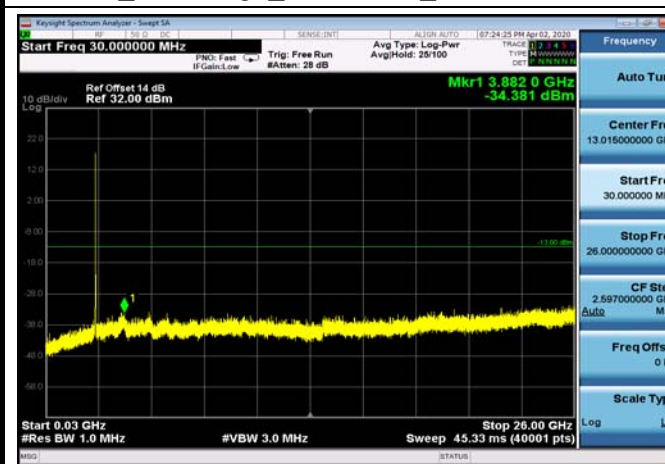
FDD7_HighRange_20+10MHz_30MHz~26GHz
