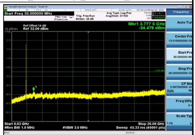
FDD7_MiddleRange_20+10MHz_30MHz~26GHz
