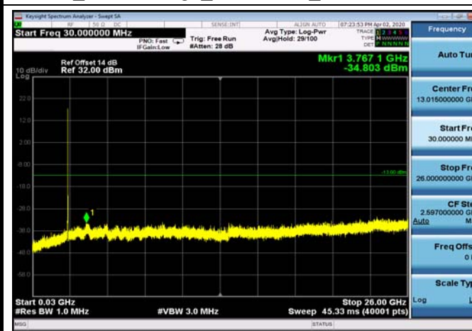
FDD7_LowRange_20+10MHz_30MHz~26GHz
