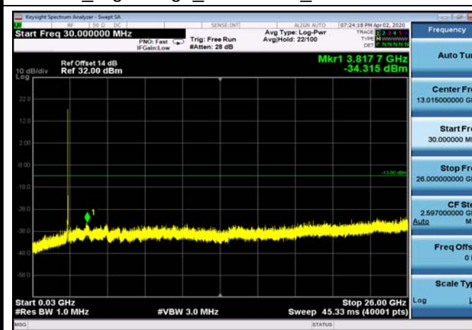
FDD7_HighRange_20+10MHz_30MHz~26GHz
