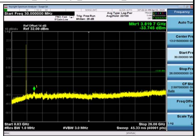
FDD7_MiddleRange_20+20MHz_30MHz~26GHz
