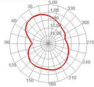
2400.000MHz H
