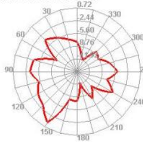
2450.000MHz E1
