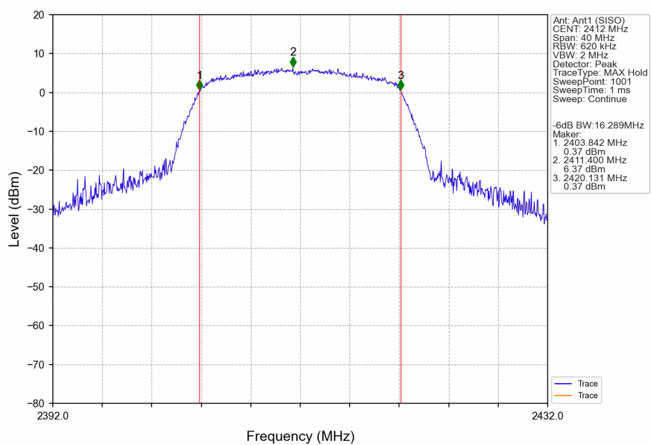
802.11g LCH 2412MHz Ant1 (SISO) NTN
