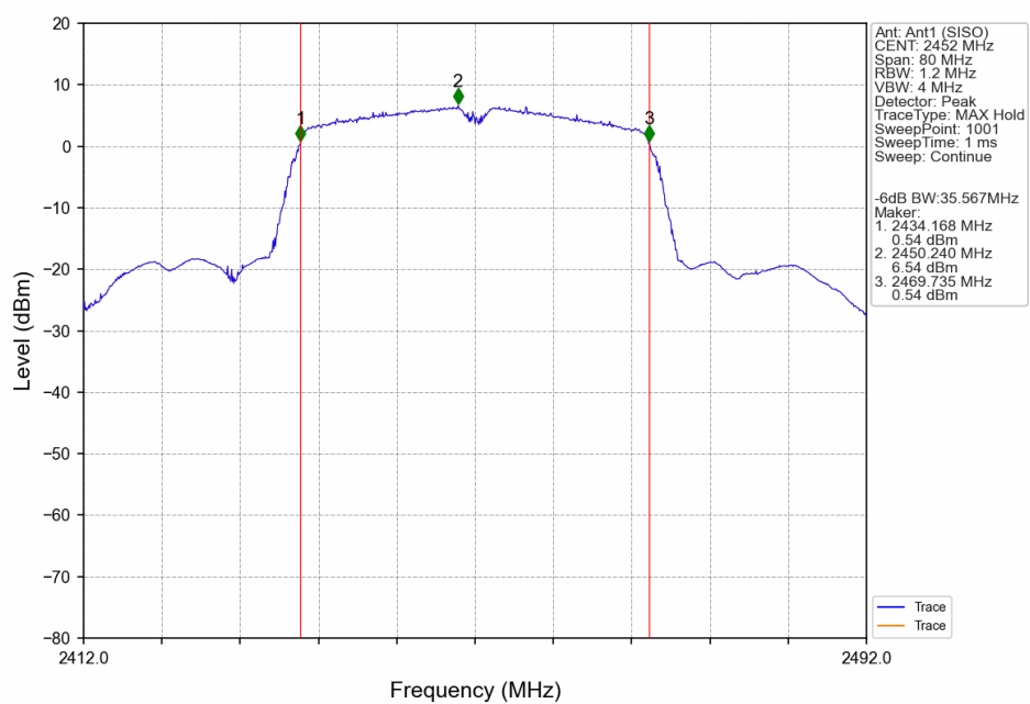
802.11n(HT40) HCH 2452MHz Ant1 (SISO) NTN
