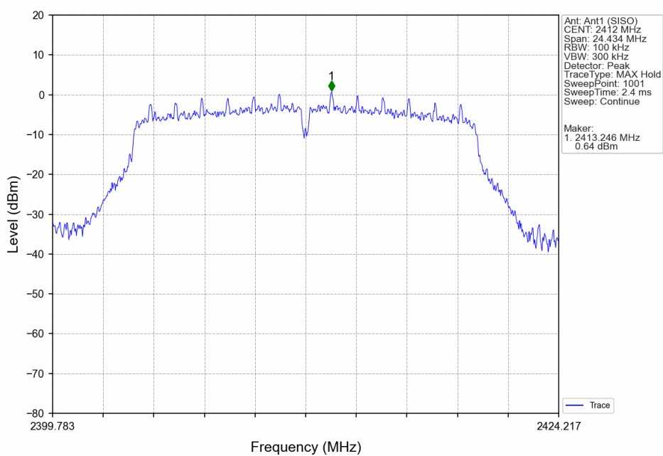
802.11g LCH 2412MHz Ant1 (SISO) NTV
