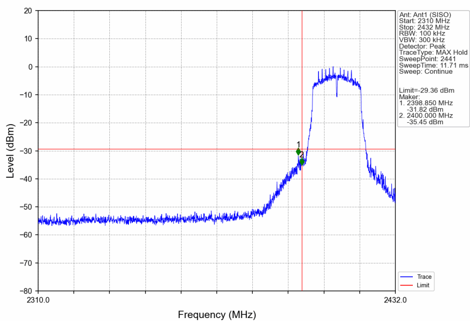
802.11g LCH 2412MHz Ant1 (SISO) NTNV
