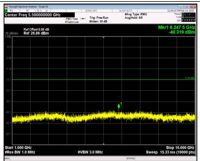
Band26-1.4MHz-QPSK-26697-1RB#0-Range2:1000~10000MHz
