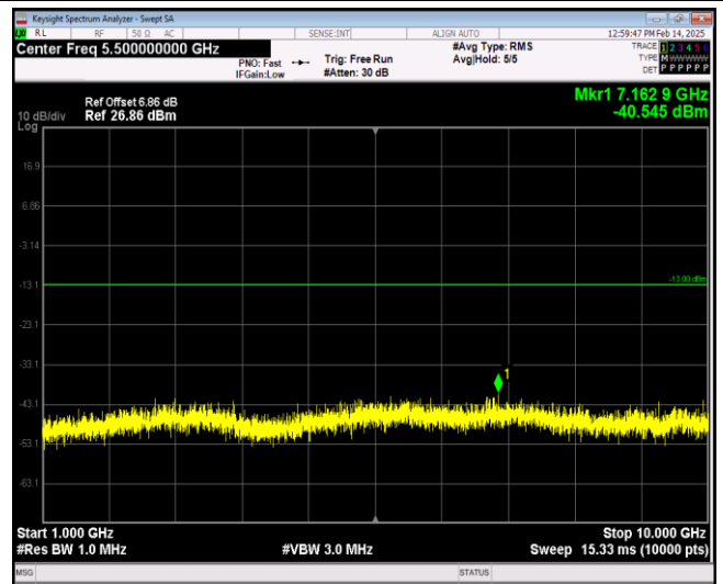
Band26-10MHz-QPSK-26740-1RB#0-Range2:1000~ 10000MHz
