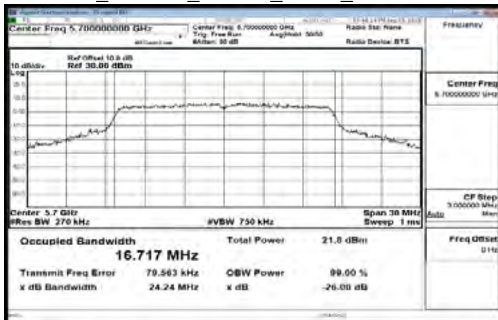
FCC_802.11a_20MHz_AUX1_5700MHz
