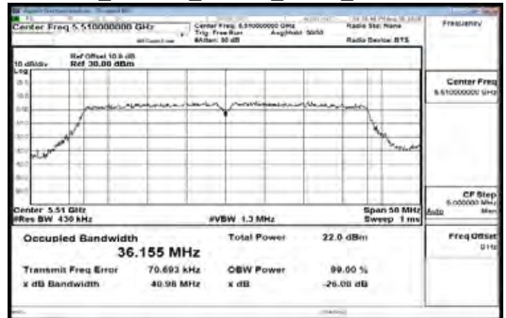
FCC_802.11n_40MHz_AUX1_5510MHz
