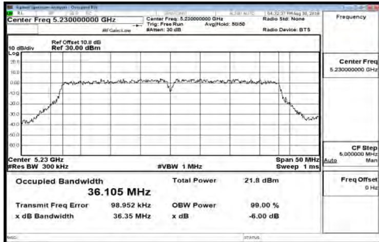
IC_802.11n_40MHz_AUX1_5230MHz
