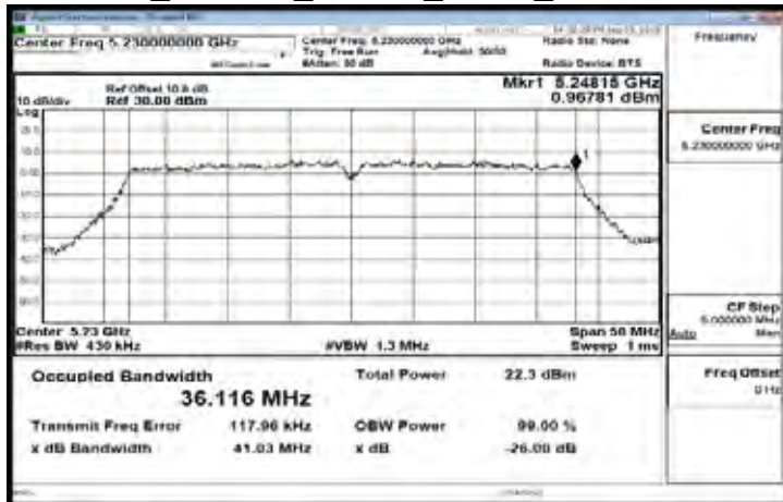
FCC_802.11n_40MHz_AUX1_5230MHz
