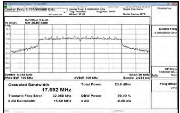
FCC_802.11n_20MHz_Main_5785MHz
