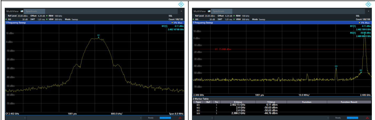
BLE 1M: Band Edge, Right Side
