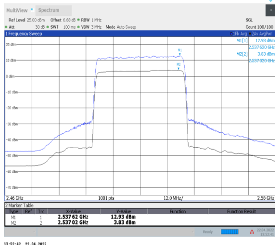
1-N7--15-40-L-1-DFT-256QAM-Outer_Full-216@0-A nt0-9.10-100%-0.00-9.10-PASS-≤13
