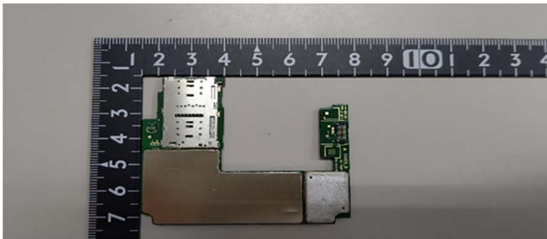
【BB PCB】
