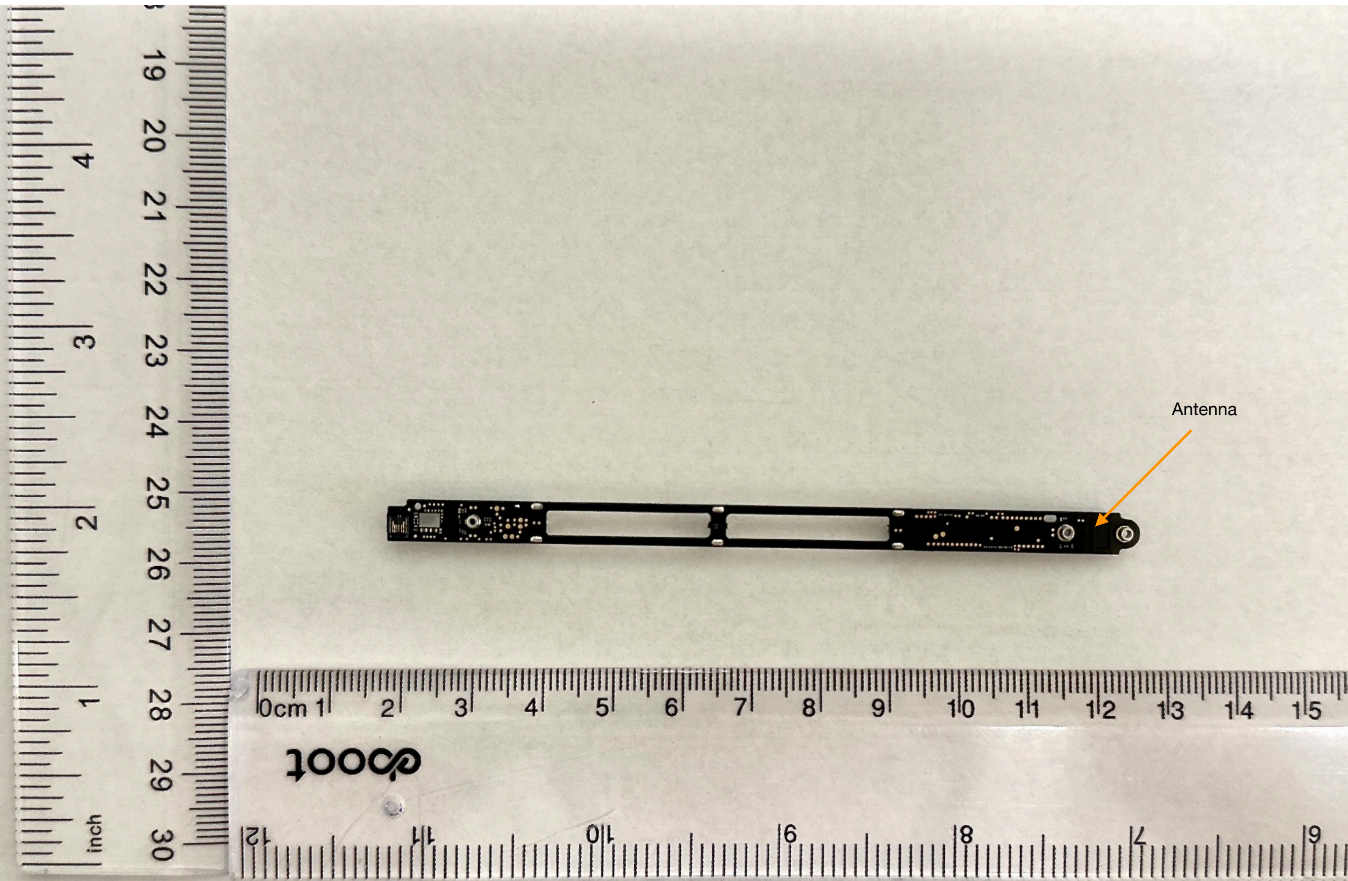
A3085 MLB PCBA - Top
