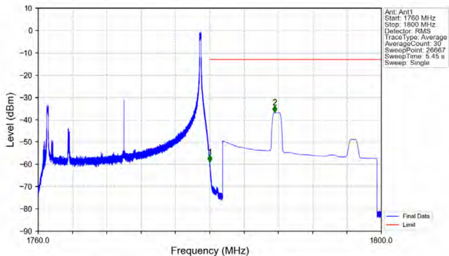
Band66_20MHz_QPSK_HCH_1770MHz_RB_1_99_NTNV
