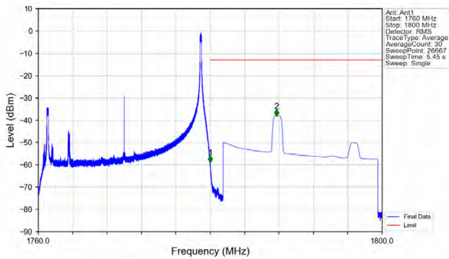
Band66_20MHz_16QAM_HCH_1770MHz_RB_1_99_NTNV
