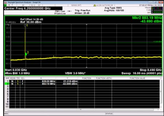
N5(5M)_DFT-s- OFDM QPSK Edge 1RB Right Mid CH
