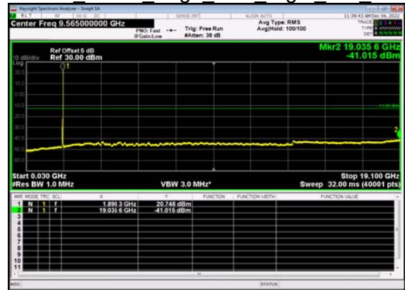
N2(20M)_DFT-s- OFDM QPSK Edge 1RB Right Mid CH
