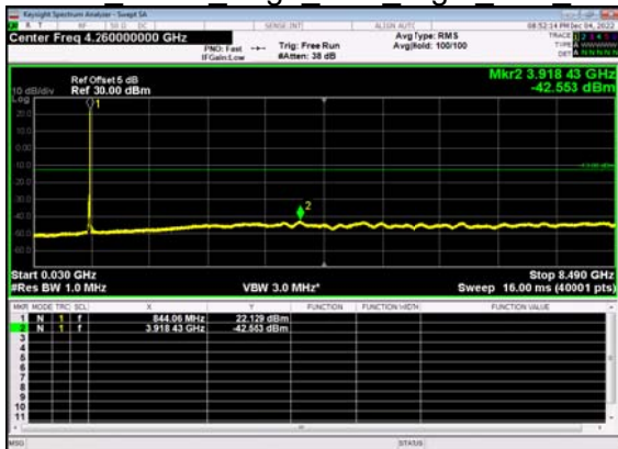
N5(20M)_DFT-s- OFDM BPSK Edge 1RB Right Low CH
