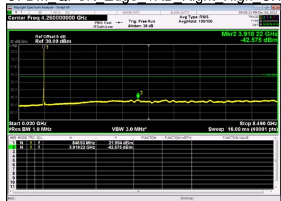
N5(20M)_DFT-s- OFDM QPSK Edge 1RB Right High CH
