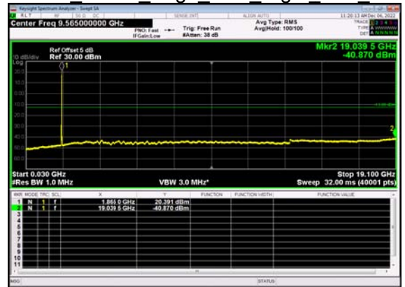
N2(15M)_DFT-s- OFDM QPSK Edge 1RB Right Low CH
