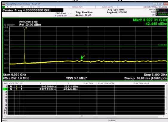
N5(20M)_DFT-s- OFDM BPSK Edge 1RB Right Mid CH
