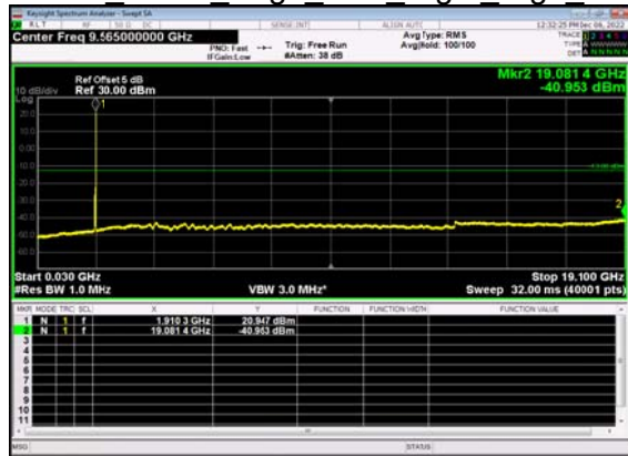
N2(20M)_DFT-s- OFDM BPSK Edge 1RB Right High CH
