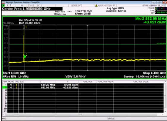
N5(5M)_DFT-s- OFDM BPSK Edge 1RB Right Mid CH
