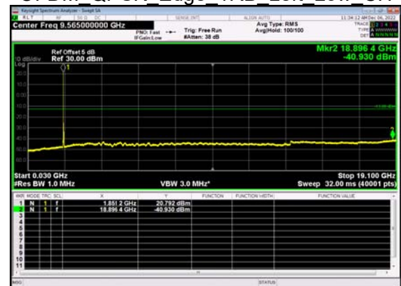
N2(20M)_DFT-s- OFDM QPSK Edge 1RB Left Low CH
