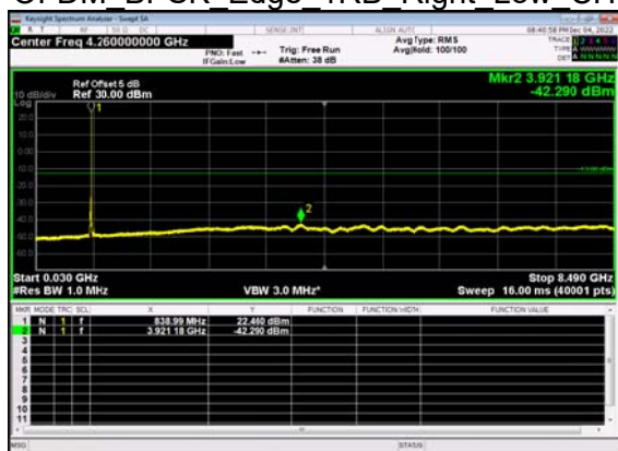
N5(15M)_DFT-s- OFDM BPSK Edge 1RB Right Low CH
