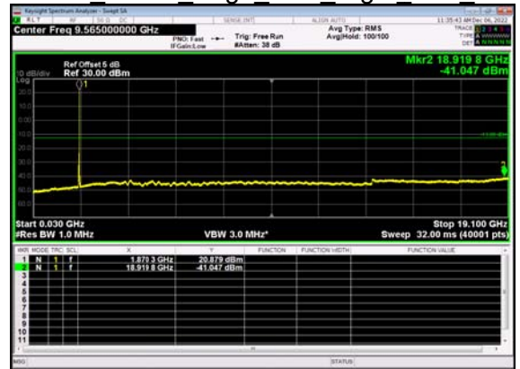
N2(20M)_DFT-s- OFDM QPSK Edge 1RB Right Low CH
