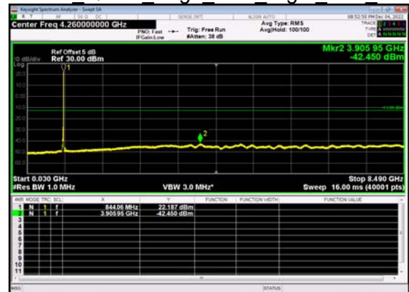
N5(20M)_DFT-s- OFDM QPSK Edge 1RB Right Low CH
