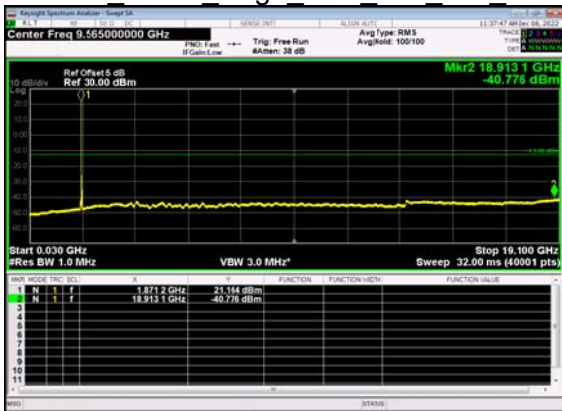
N2(20M)_DFT-s- OFDM BPSK Edge 1RB Left Mid CH
