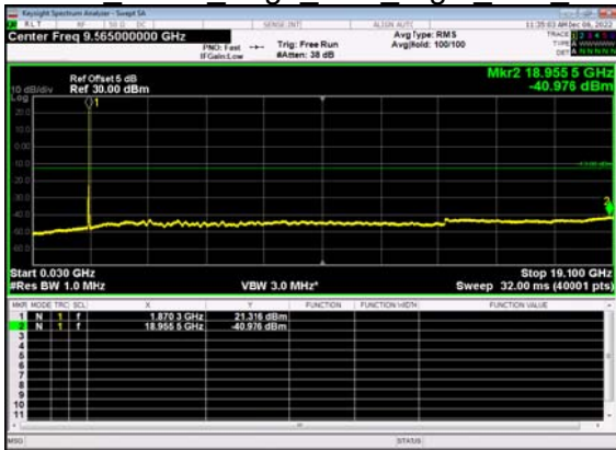
N2(20M)_DFT-s- OFDM BPSK Edge 1RB Right Low CH
