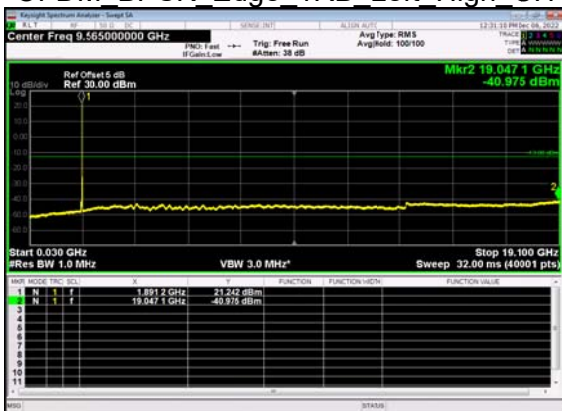
N2(20M)_DFT-s- OFDM BPSK Edge 1RB Left High CH
