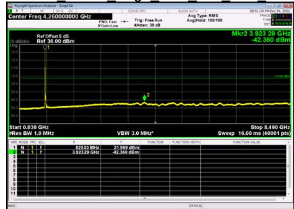
N5(20M)_DFT-s- OFDM QPSK Edge 1RB Left Low CH
