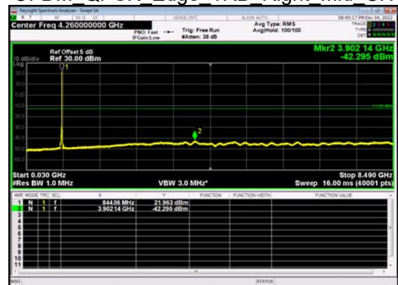
N5(15M)_DFT-s- OFDM QPSK Edge 1RB Right Mid CH
