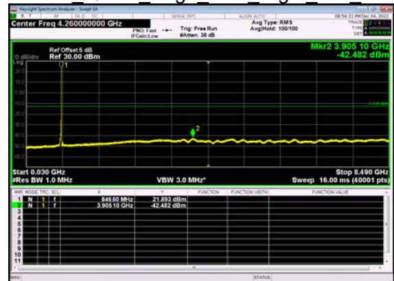
N5(20M)_DFT-s- OFDM QPSK Edge 1RB Right Mid CH
