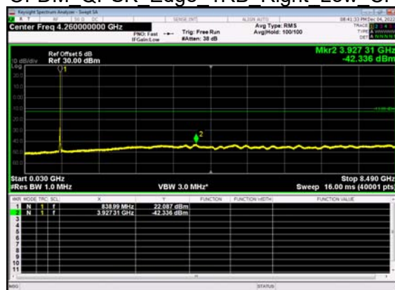
N5(15M)_DFT-s- OFDM QPSK Edge 1RB Right Low CH
