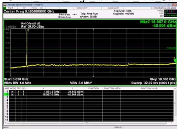
N2(20M)_DFT-s- OFDM BPSK Edge 1RB Left Low CH
