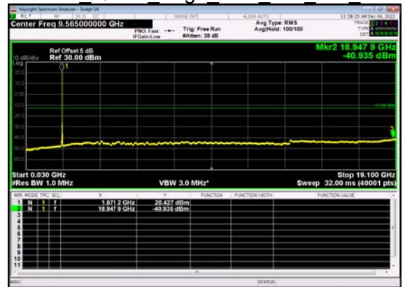
N2(20M)_DFT-s- OFDM QPSK Edge 1RB Left Mid CH
