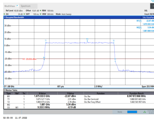
Band2-10MHz-16QAM-18900-50RB#0
