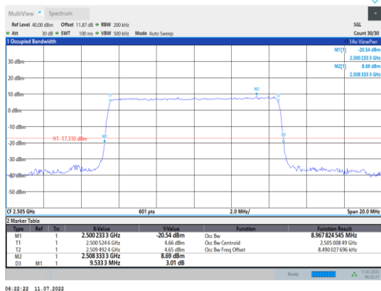
Band7-10MHz-QPSK-20800-50RB#0
