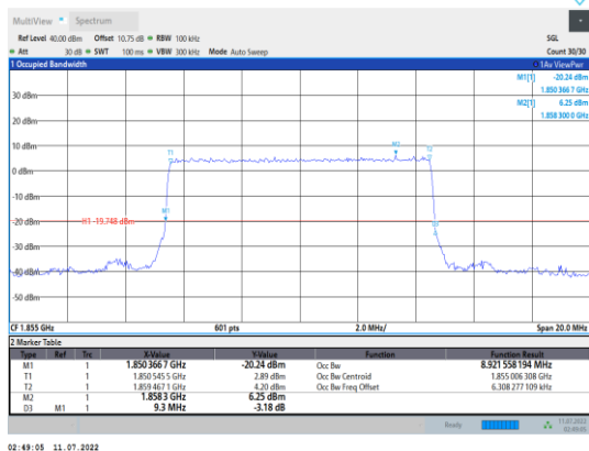
Band2-10MHz-QPSK-18650-50RB#0
