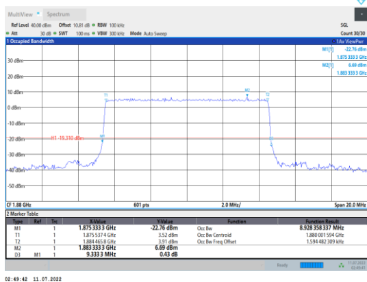
Band2-10MHz-QPSK-18900-50RB#0
