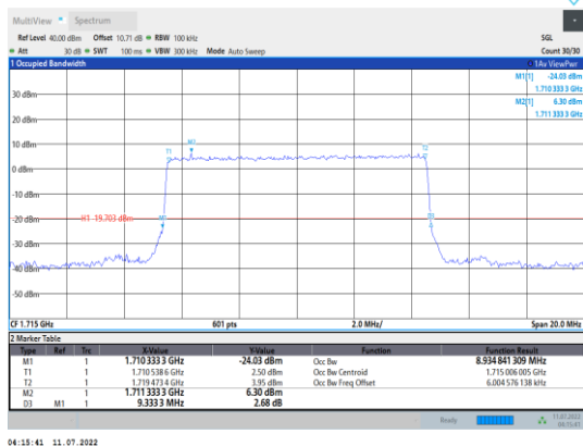
Band4-10MHz-QPSK-20000-50RB#0
