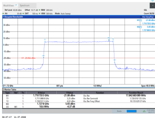
Band4-20MHz-QPSK-20050-100RB#0
