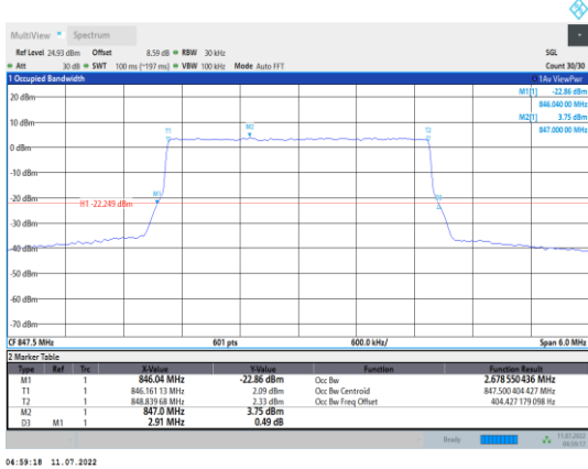
Band5-3MHz-QPSK-20635-15RB#0
