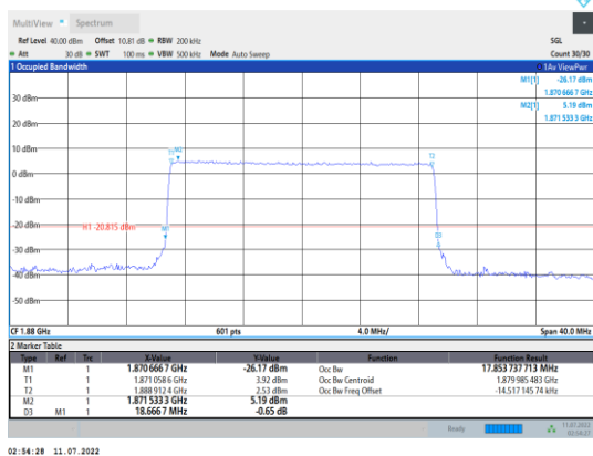
Band2-20MHz-QPSK-18900-100RB#0
