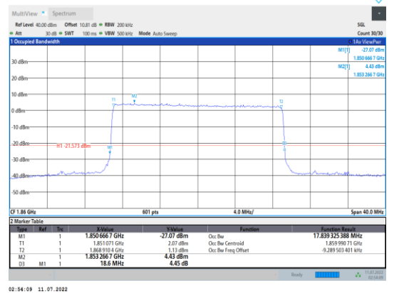
Band2-20MHz-16QAM-18700-100RB#0
