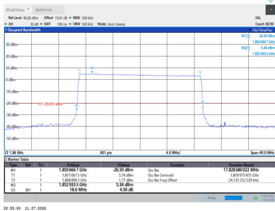
Band2-20MHz-QPSK-18700-100RB#0
