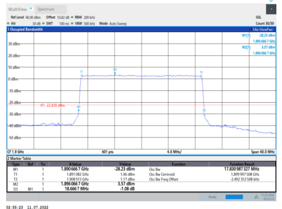
Band2-20MHz-16QAM-19100-100RB#0
