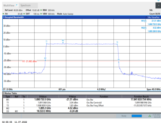
Band2-20MHz-QPSK-19100-100RB#0
