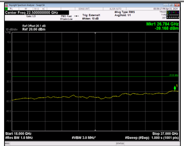
Band41_20MHz_64QAM_41490_1RB#0_18000~27000_1 8000~27000
