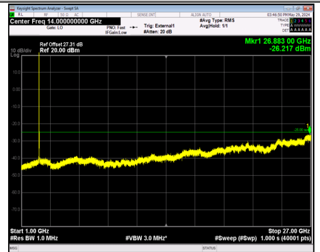
Band38_20MHz_64QAM_38000_1RB#0_1000~27000_10 00~27000
