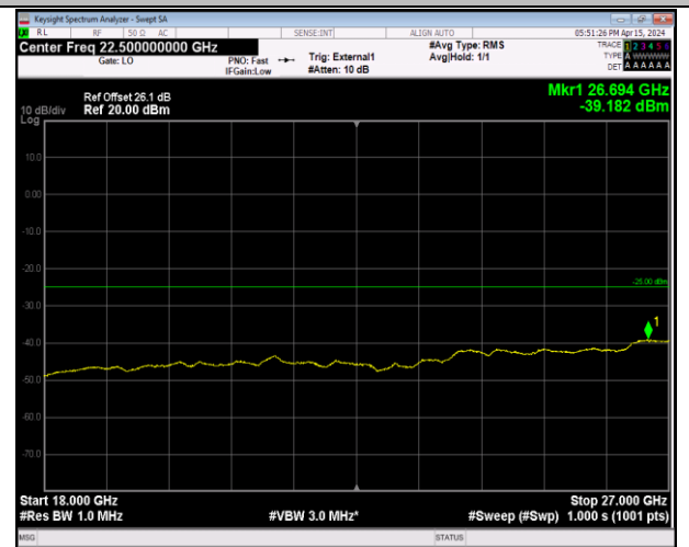
Band41_20MHz_QPSK_39750_1RB#0_18000~27000_18 000~27000
