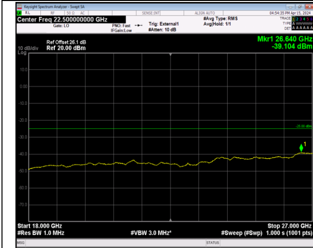
Band41_5MHz_16QAM_40620_1RB#0_18000~27000_18 000~27000
