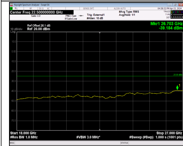
Band41_5MHz_64QAM_41565_1RB#0_18000~27000_18 000~27000
