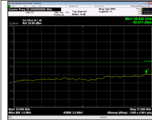
Band41_20MHz_16QAM_39750_1RB#0_18000~27000_1 8000~27000
