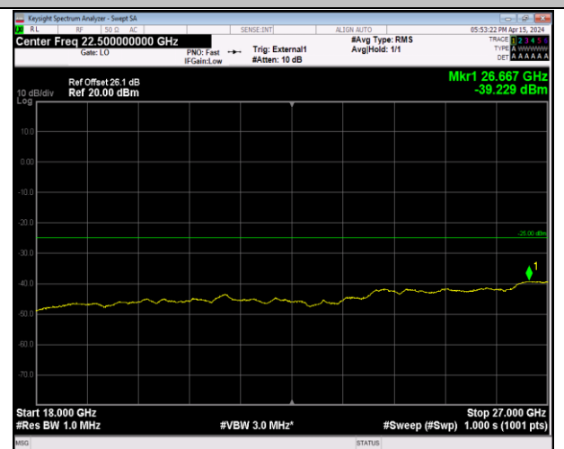
Band41_20MHz_64QAM_39750_1RB#0_18000~27000_1 8000~27000
