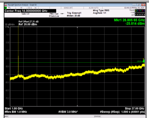
Band38_20MHz_64QAM_38150_1RB#0_1000~27000_10 00~27000
