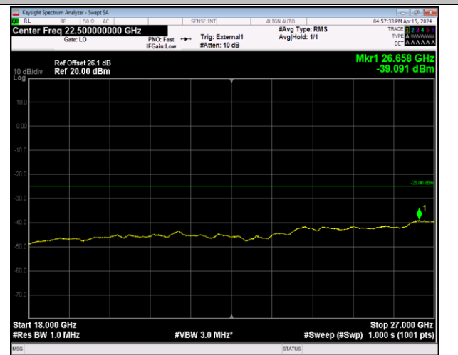
Band41_5MHz_16QAM_41565_1RB#0_18000~27000_18 000~27000
