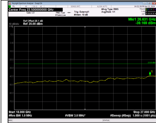
Band41_5MHz_64QAM_39675_1RB#0_18000~27000_18 000~27000
