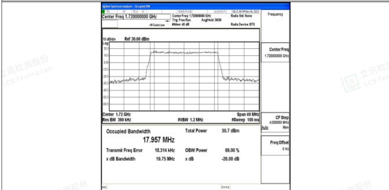
Band4-20MHz-QPSK-20050-100RB#0-PASS
