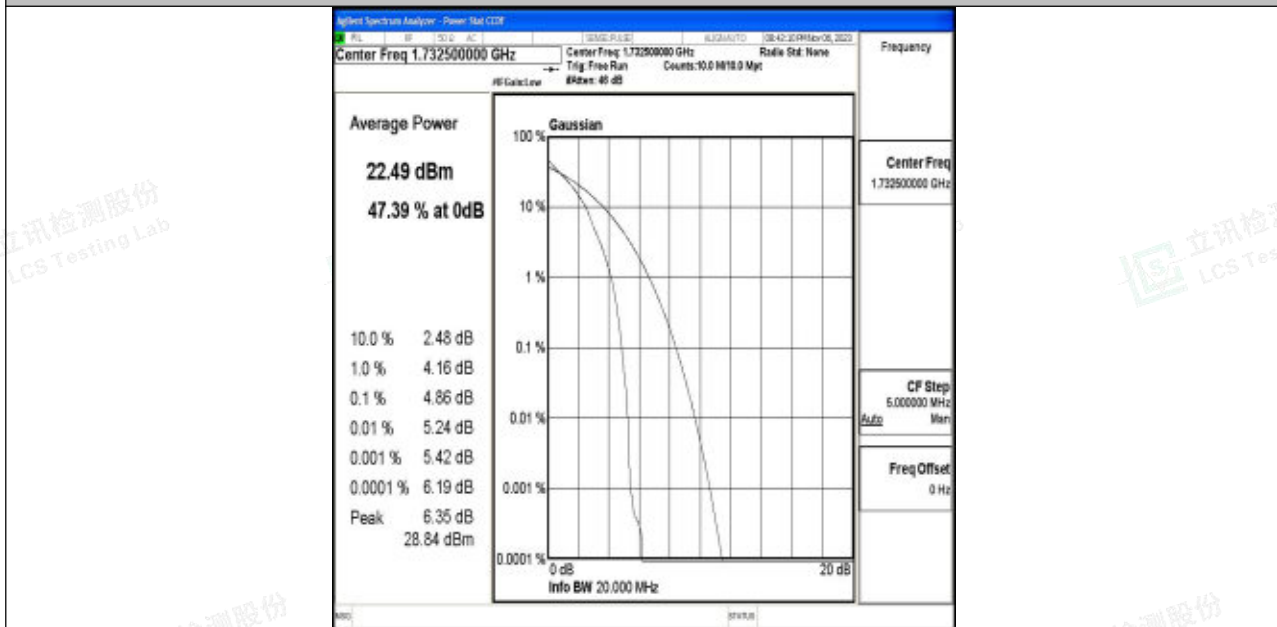
Band4-20MHz-QPSK-20175-1RB#0-PASS
