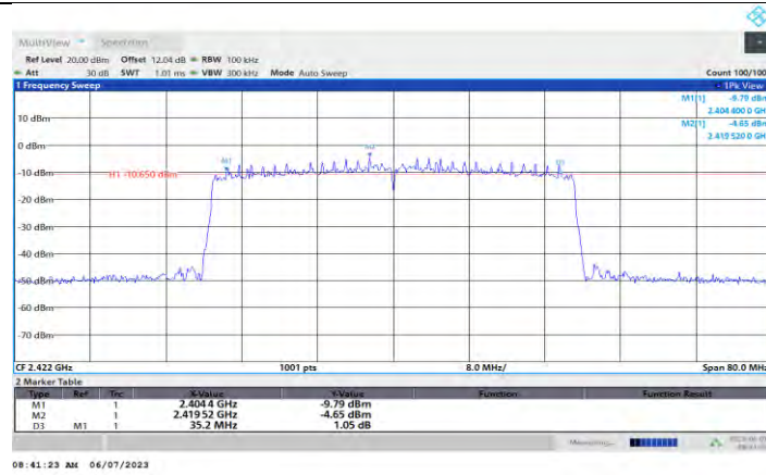
11AX40MIMO_Ant1_2422
