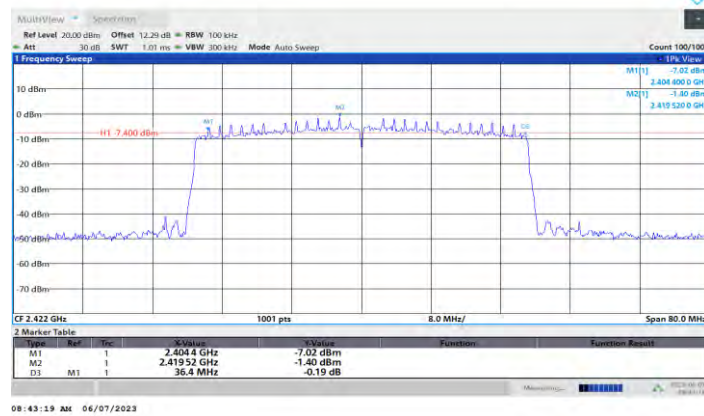
11AX40MIMO_Ant2_2422
