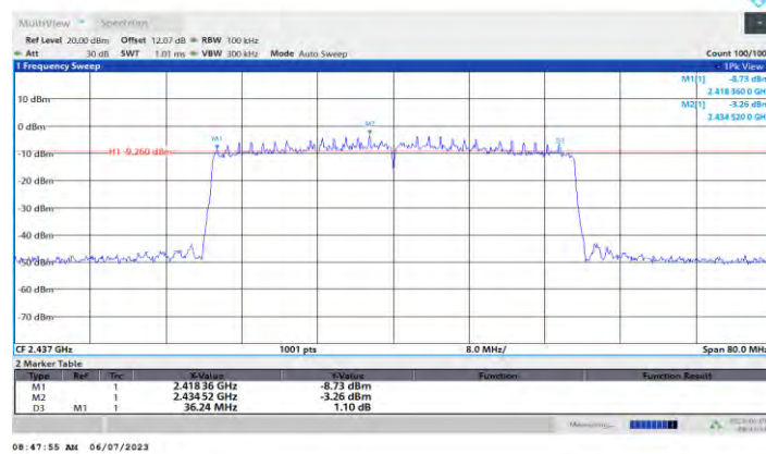
11AX40MIMO_Ant1_2437
